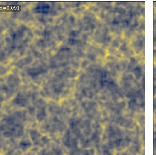
cnn volcanic-plasma-59
