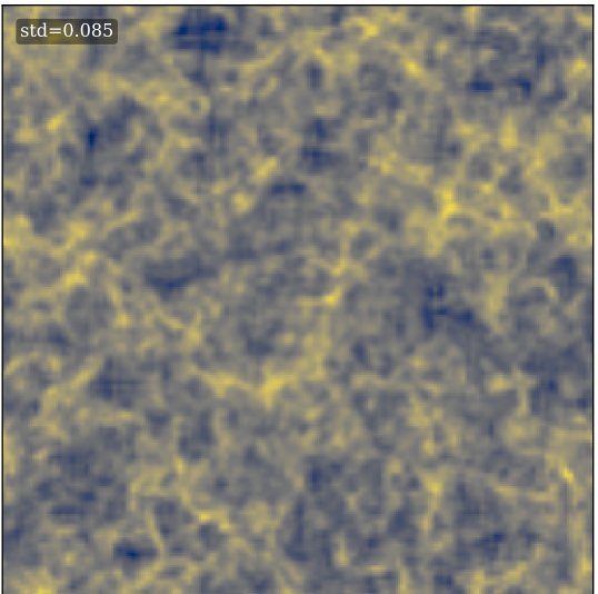
cnn lemon-cloud-74
