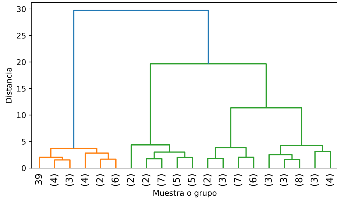
Dendrograma (Ward)
