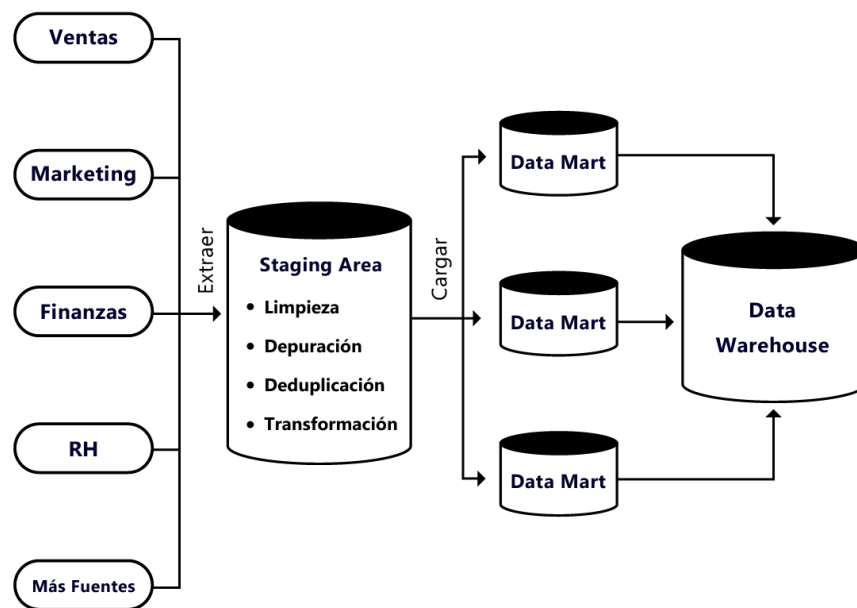
Figura 7.1.: Enfoque Kimball para construcción de Data Warehouse
