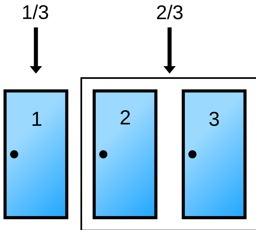
Figura 119.1.: Notemos como la probabilidad de encontrar el auto detrás de las puertas cerradas es de \frac{1}{3} , mientras que la probabilidad de encontrar la cabra es de \frac{2}{3}
