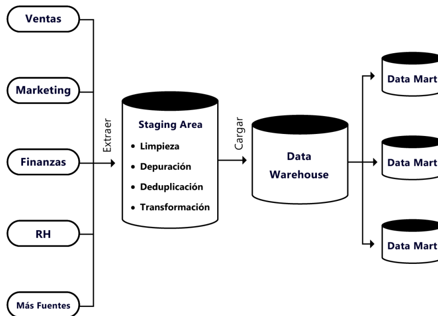
Figura 7.2.: Enfoque Inmon para construcción de Data Warehouse
