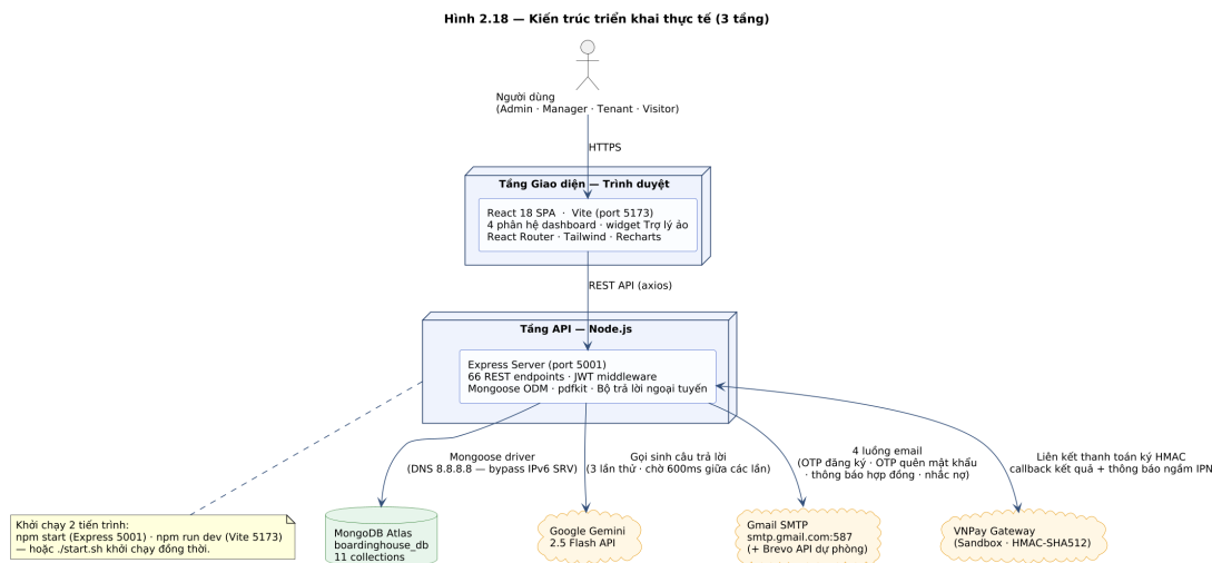
Hình 2.18. Sơ đồ kiến trúc triển khai thực tế 3 tầng
