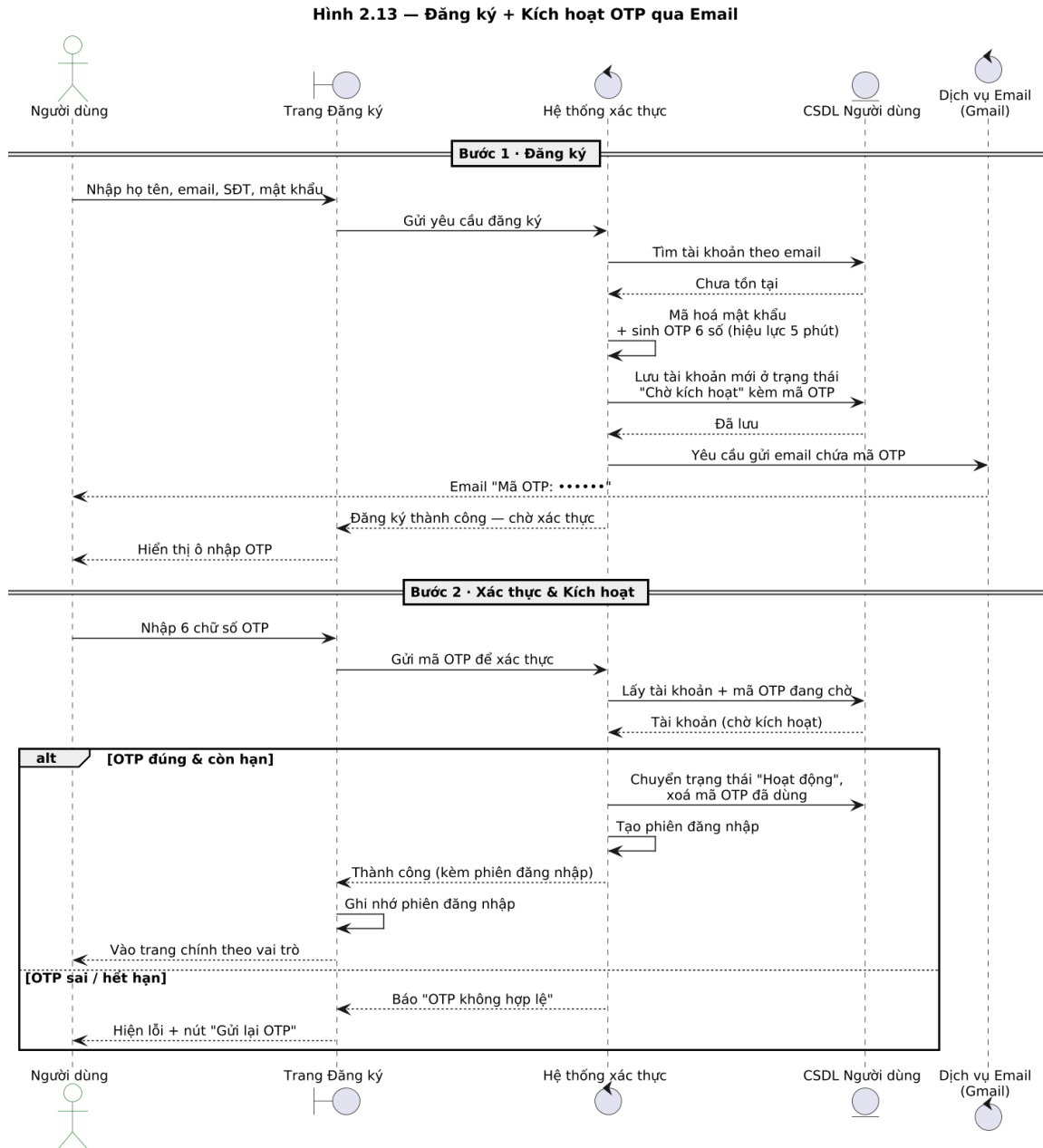
Hình 2.13. Sơ đồ tuần tự UC Đăng ký tài khoản & Kích hoạt OTP qua Email
