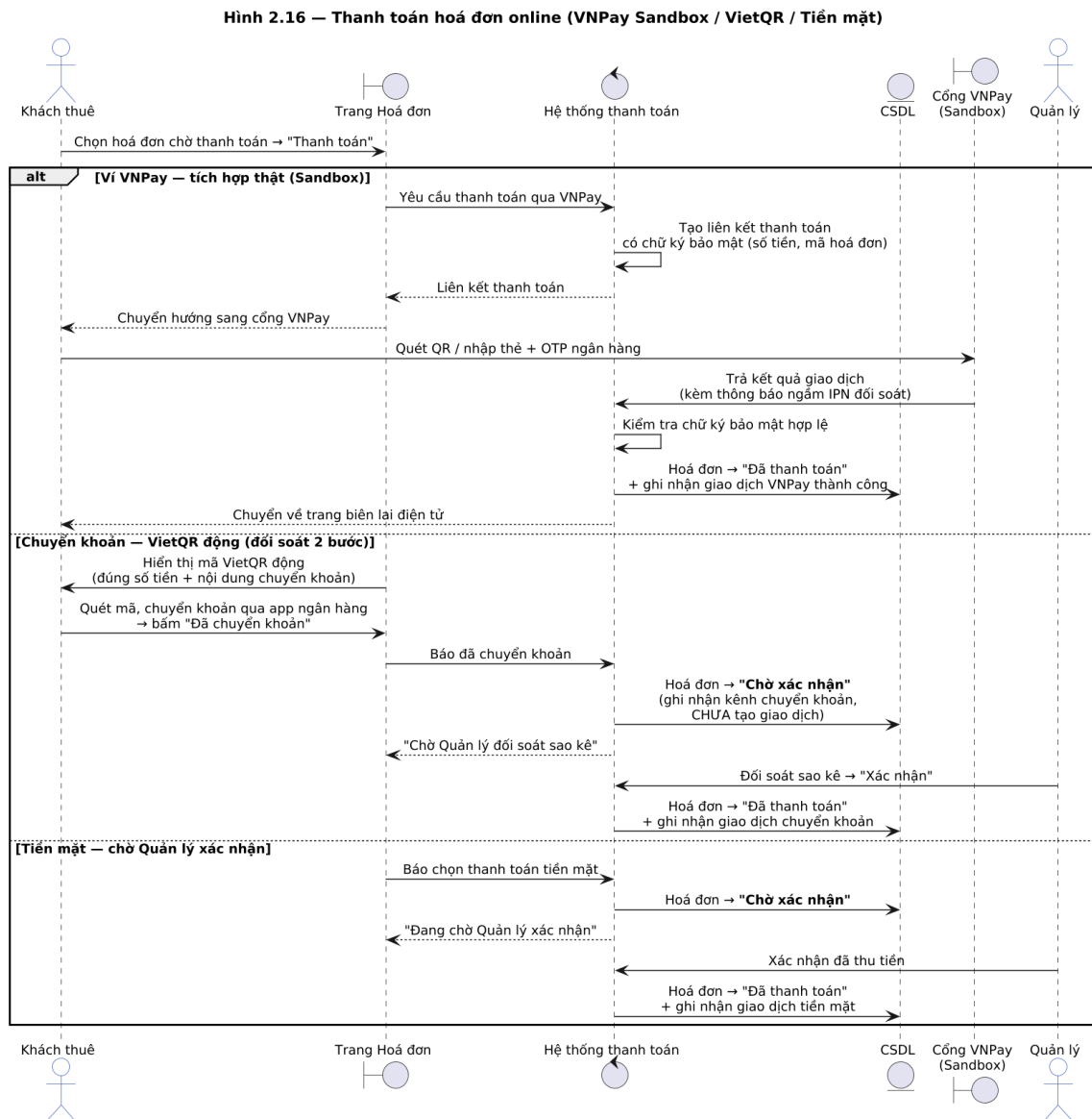
Hình 2.16. Sơ đồ tuần tự UC Thanh toán hoá đơn online (VNPAY Sandbox thật / VietQR chuyển khoản)
