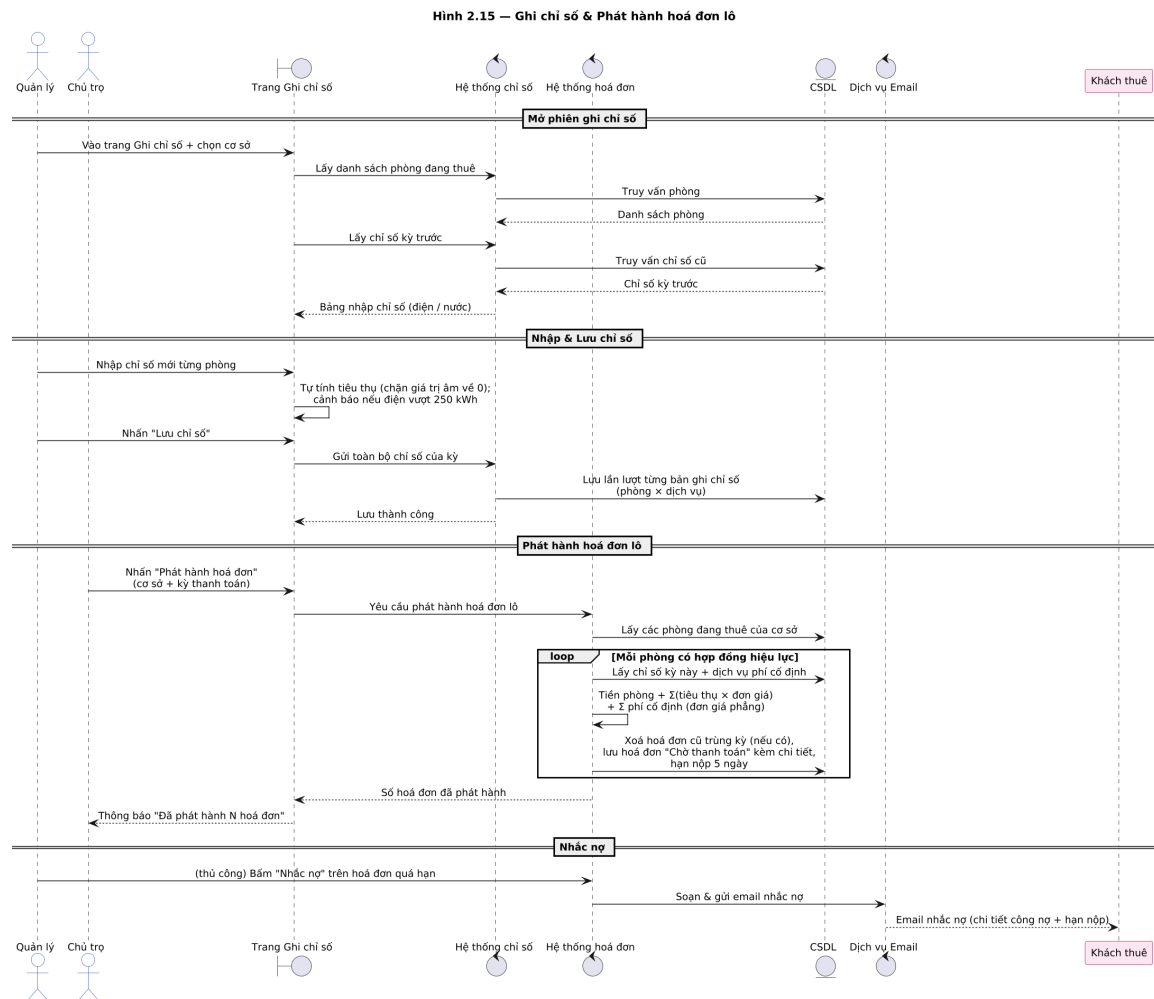
Hình 2.15. Sơ đồ tuần tự UC Ghi chỉ số & tạo hoá đơn
