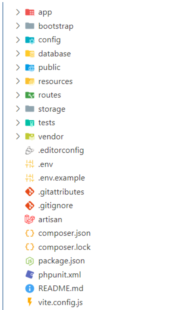
Hình 2.2 Cấu trúc thư mục trong Laravel
