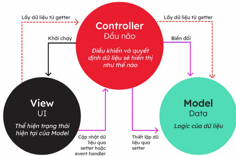
Hình 2.1 Kiến trúc MVC
