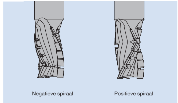
Rechte snijhoek snede, spiraalvormig geplaatst
