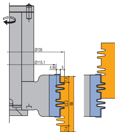
Verlijmprofiel positief, houtdikte 68 mm
