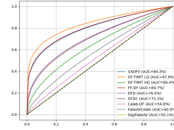
(a) Meso4
