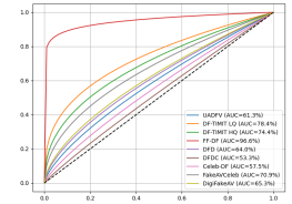
(d) Capsule
