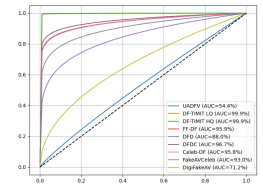
(h) SFConv
