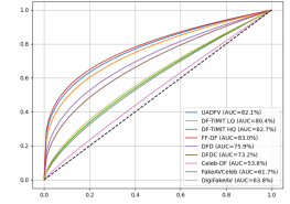
(b) MesoInception4
