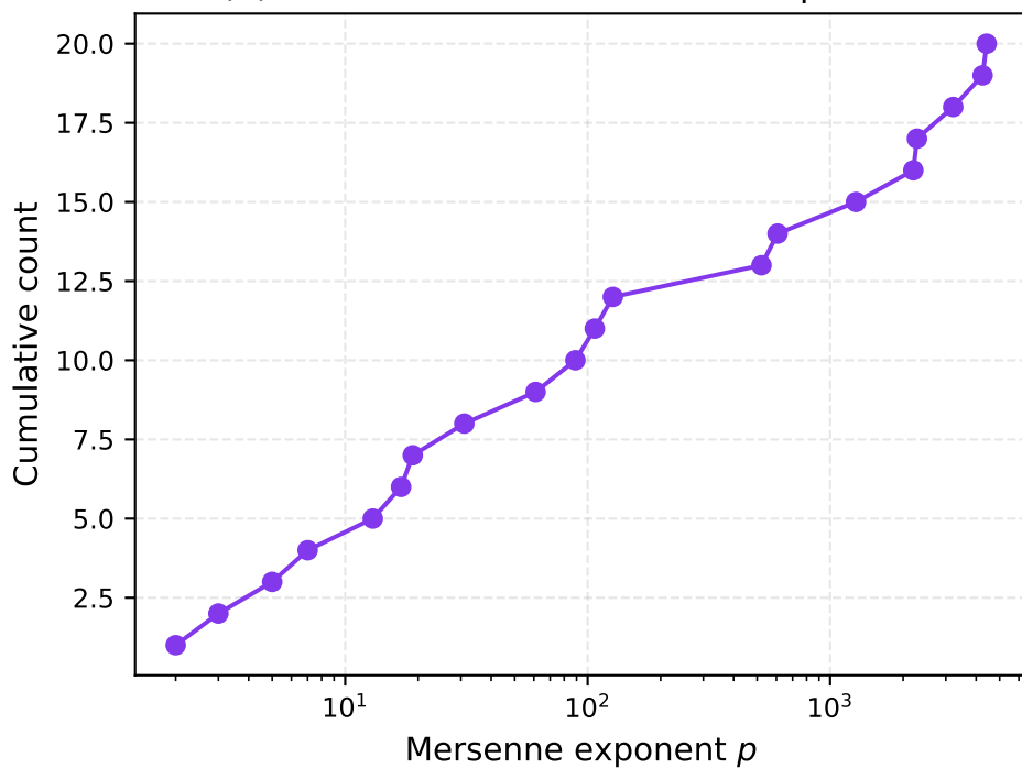
(d) Cumulative Distribution of Exponents
