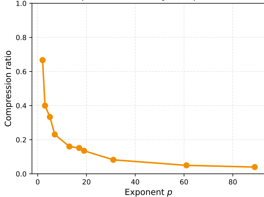
(d) Binary Structure of Perfect Numbers
