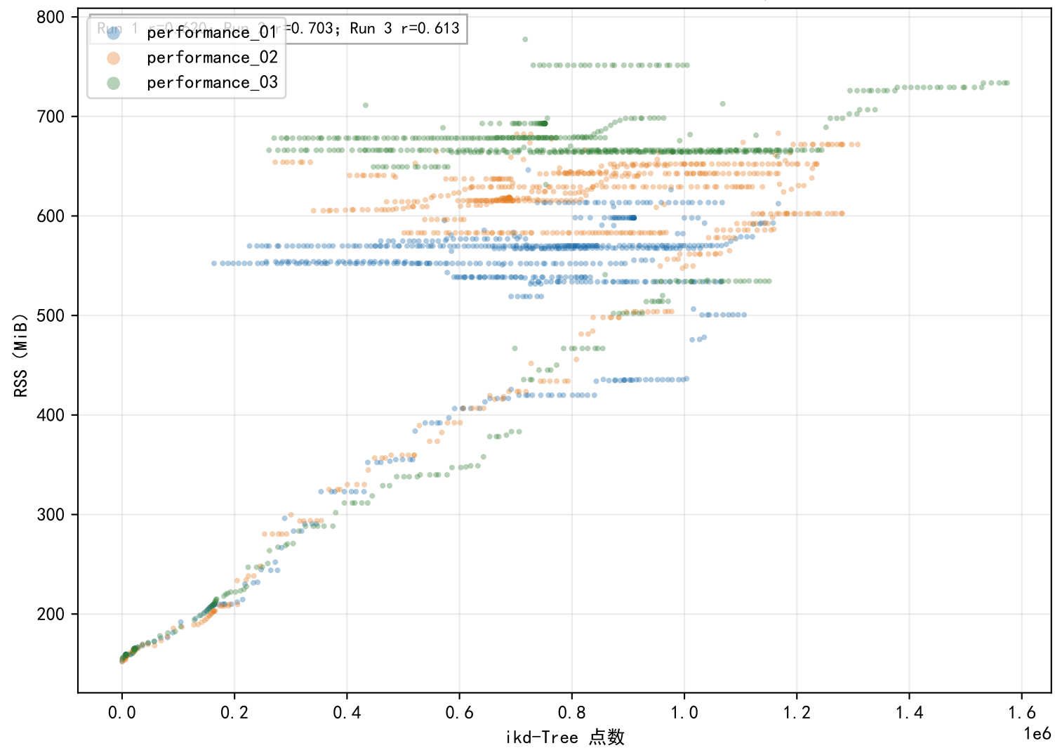
AMtown01 RSS 与 ikd-Tree 点数关系（墙钟时间对齐，仅相关性）
