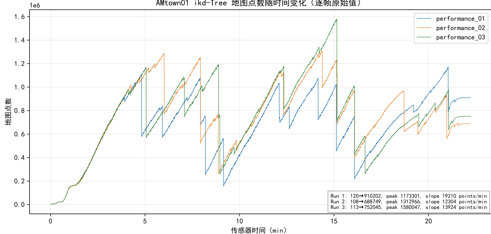
AMtown01 ikd-Tree 地图点数随时间变化 (逐帧原始值)
