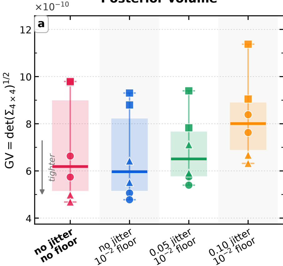
Posterior volume
