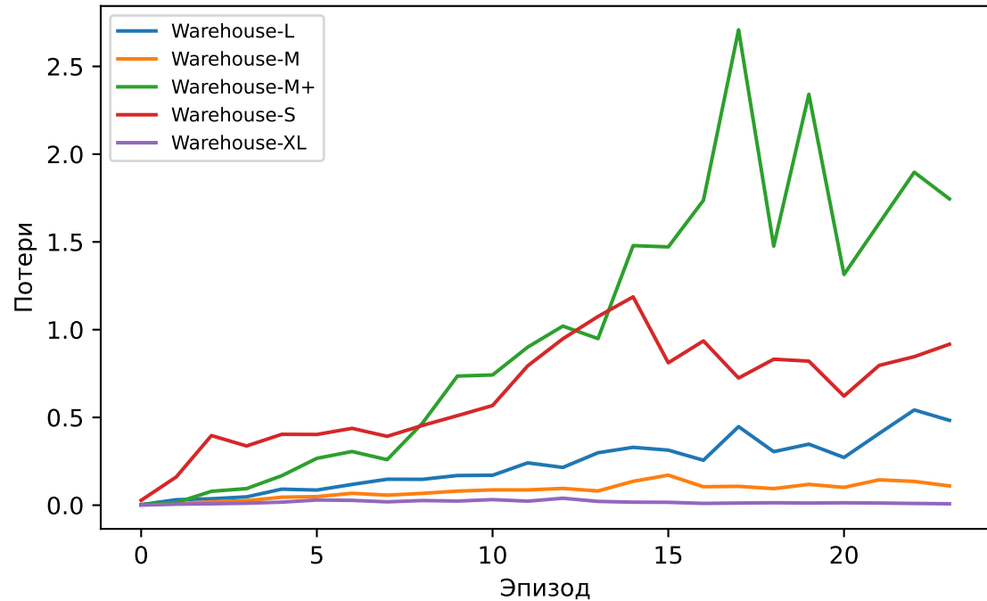
Потери QMIX
