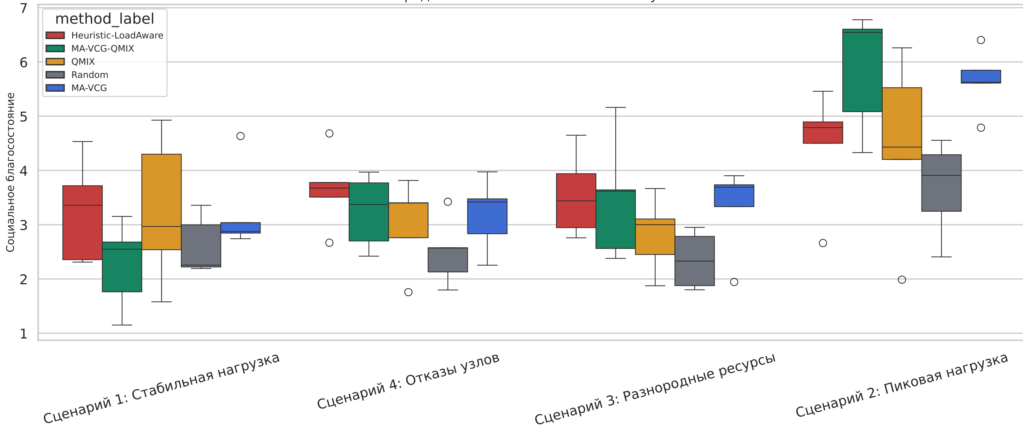
Распределение SW по независимым запускам
