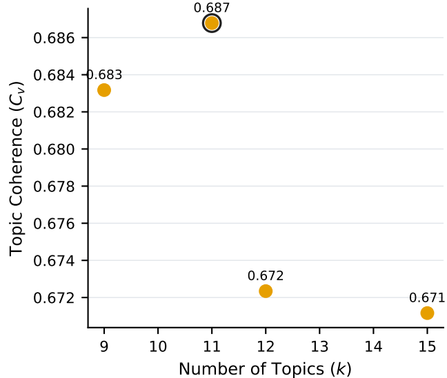
(b) NMF
