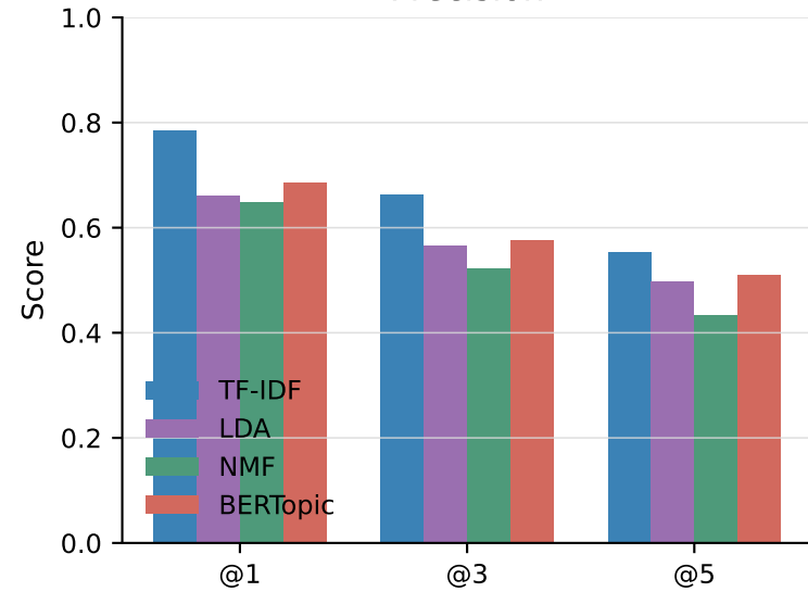
Precision
