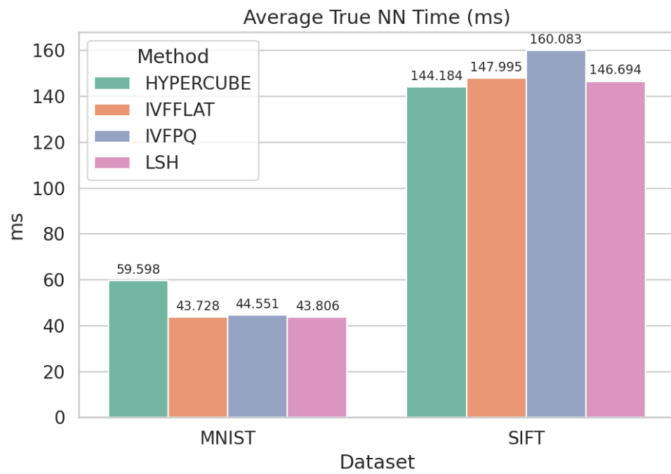
Εικόνα 35: Διάγραμμα t_{True} με πλήρη δεδομένα
