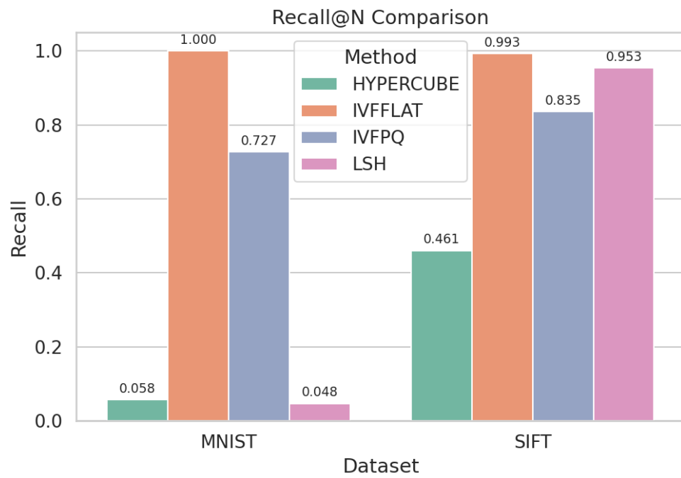
Εικόνα 32: Διάγραμμα Recall με πλήρη δεδομένα
