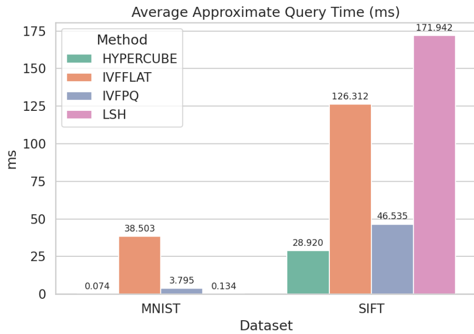
Εικόνα 34: Διάγραμμα t_{Approximate} με πλήρη δεδομένα
