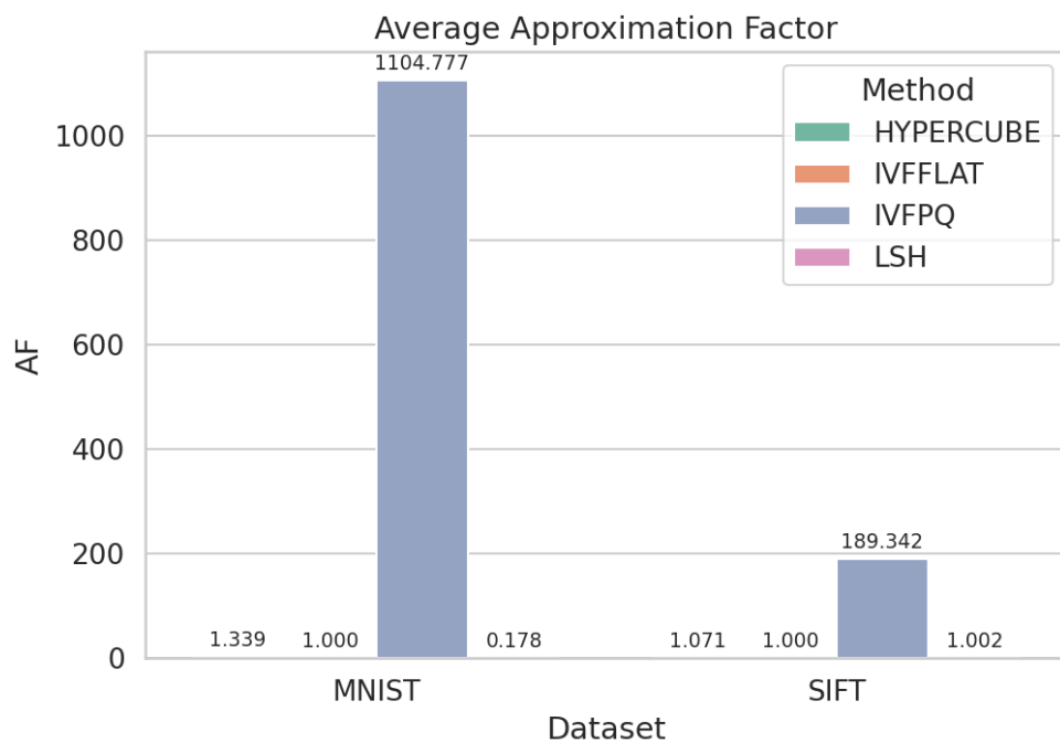
Εικόνα 31: Διάγραμμα AF με πλήρη δεδομένα
