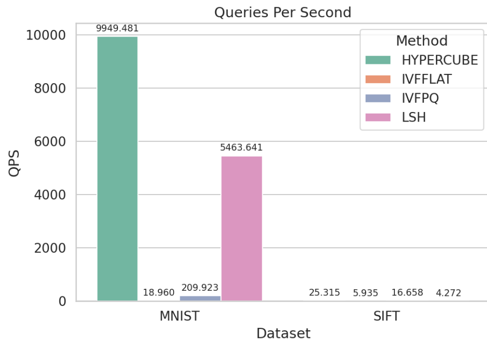
Εικόνα 33: Διάγραμμα QPS με πλήρη δεδομένα
