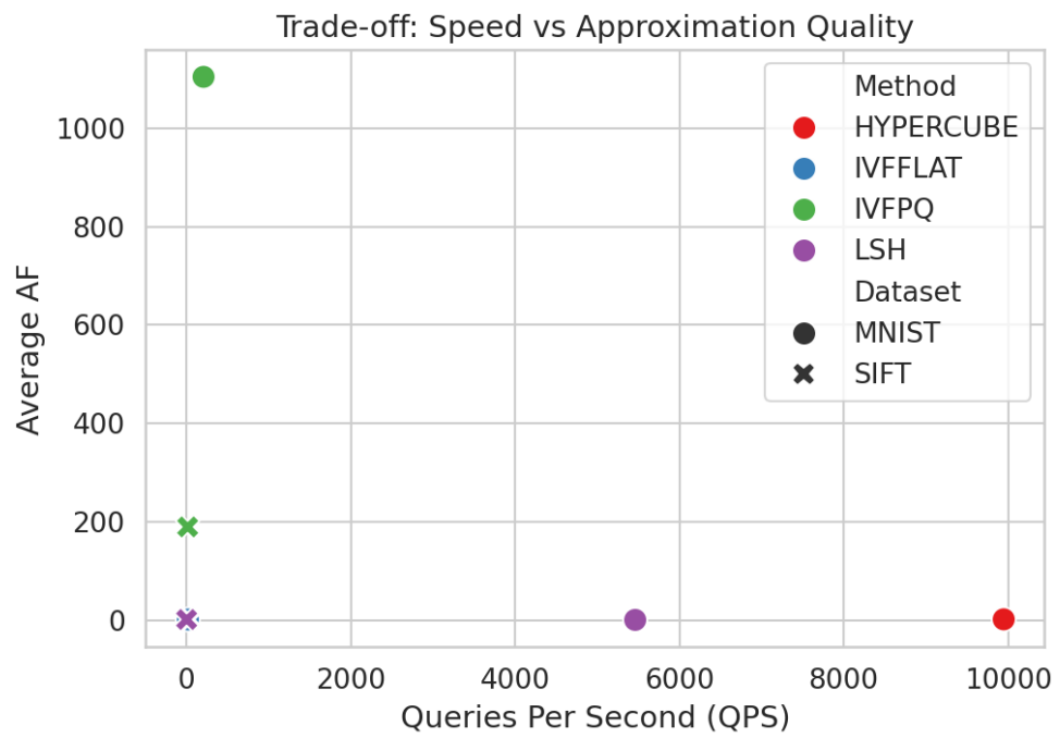
Εικόνα 36: Διάγραμμα Trade-off με πλήρη δεδομένα
