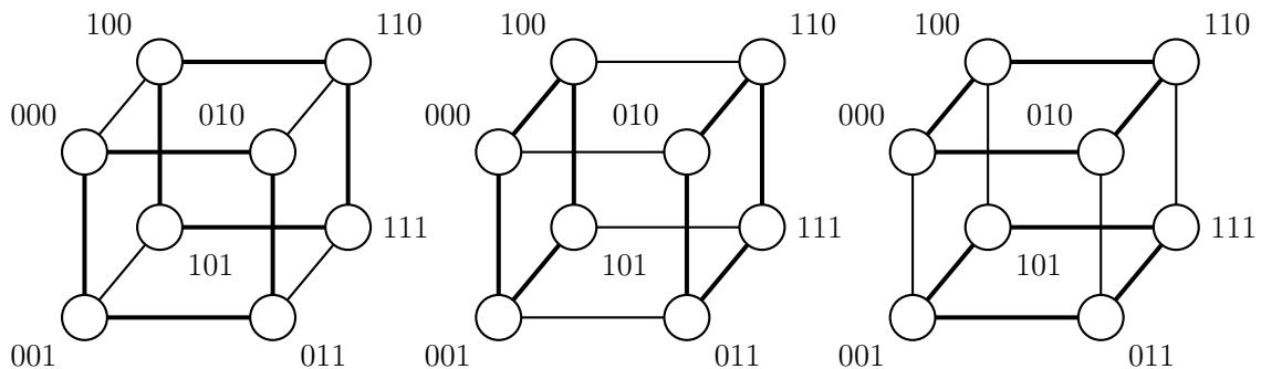
Σχήμα 20: Τρεις διακριτές διαμερίσεις ενός τριδιάστατου υπερκύβου σε δύο διδιάστατους κύβους. Οι σύνδεσμοι που συνδέουν επεξεργαστές μέσα σε μία διαμέριση υποδεικνύονται με έντονες γραμμές.
