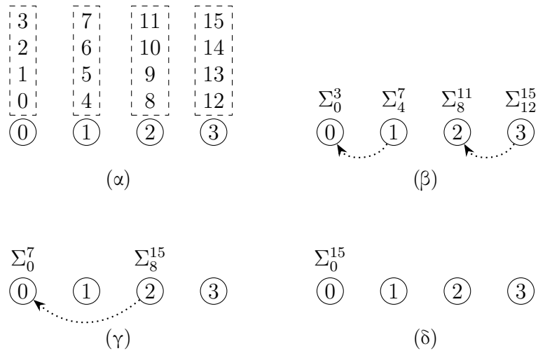
Σχήμα 30: Ένας βέλτιστος ως προς το κόστος τρόπος υπολογισμού του αθροίσματος 16 αριθμών σε έναν υπερκύβο τεσσάρων επεξεργαστών.
