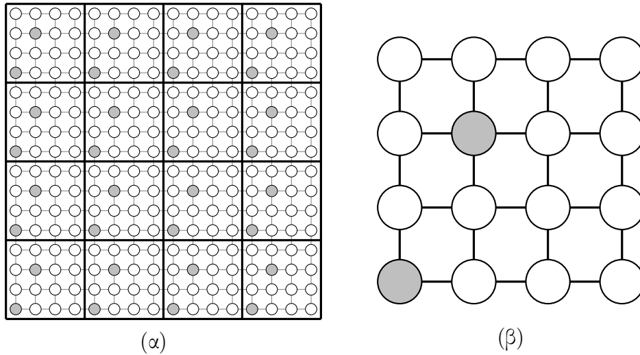
Σχήμα 54: Απεικόνιση του γραφήματος πλέγματος (α) σε ένα πλέγμα (β) χρησιμοποιώντας την κυκλική απεικόνιση σκακιέρας. Σε αυτό το παράδειγμα, n = 16 και \sqrt{p} = 4 . Οι σκιασμένες κορυφές απεικονίζονται στους αντίστοιχους σκιασμένους επεξεργαστές πλέγματος.
