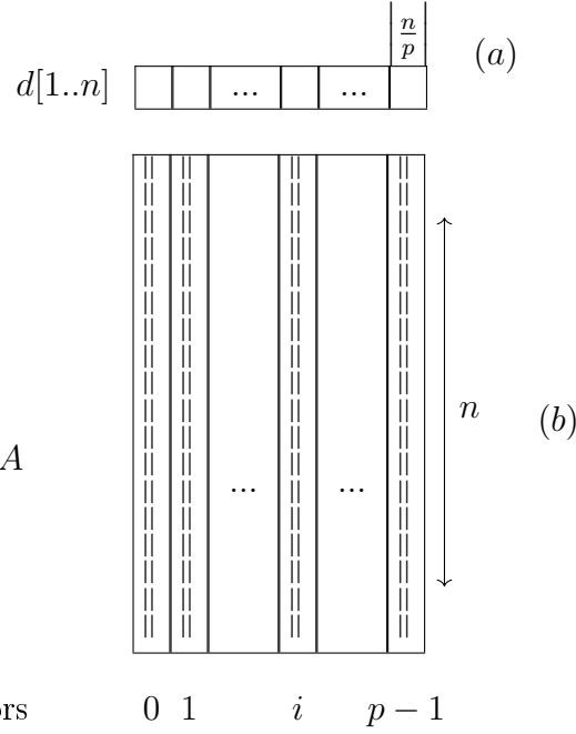
Σχήμα 36: Η διαμέριση του πίνακα απόστασης d και ο πίνακας γειτνίασης A μεταξύ p επεξεργαστών.
