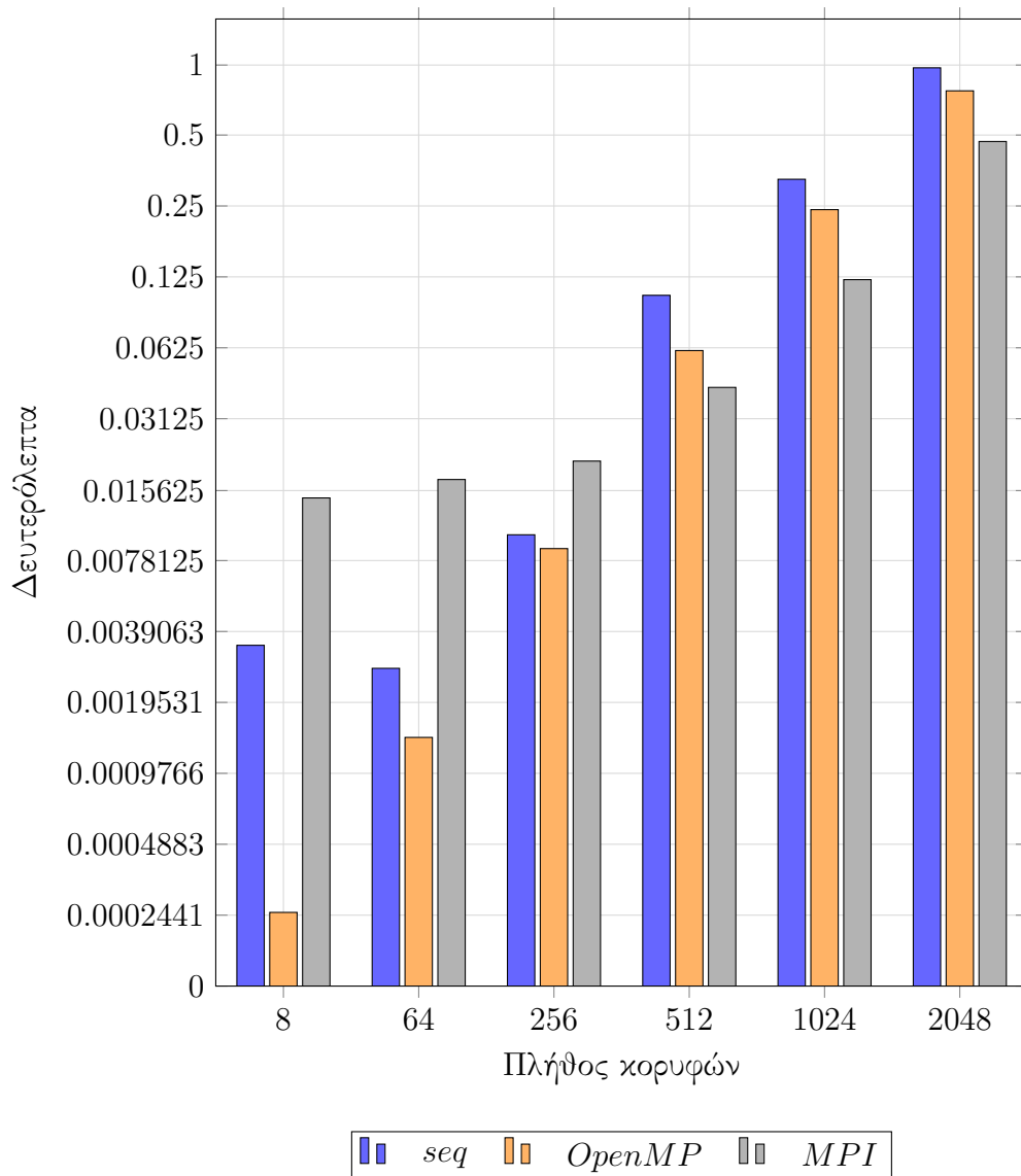
Σχήμα 37: Ο καλύτερος χρόνος εκτέλεσης για κάθε υλοποίηση σε διαφορετικά σύνολα δεδομένων
