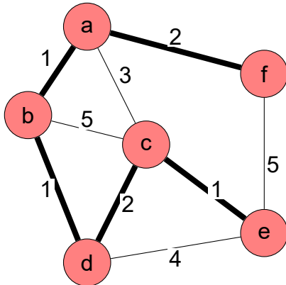
Σχήμα 36: Ο αλγόριθμος του Prim
