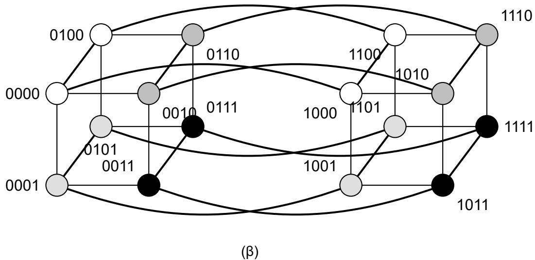
Σχήμα 21: Οι διδιάστατοι υποκύβοι ενός τετραδιάστατου υπερκύβου που προκύπτουν με σταθεροποίηση των δύο σημαντικότερων ψηφίων ετικέτας (α) και των δύο λιγότερο σημαντικών ψηφίων ετικέτας (β). Οι επεξεργαστές μέσα σε έναν υποκύβο συνδέονται με έντονες γραμμές.
