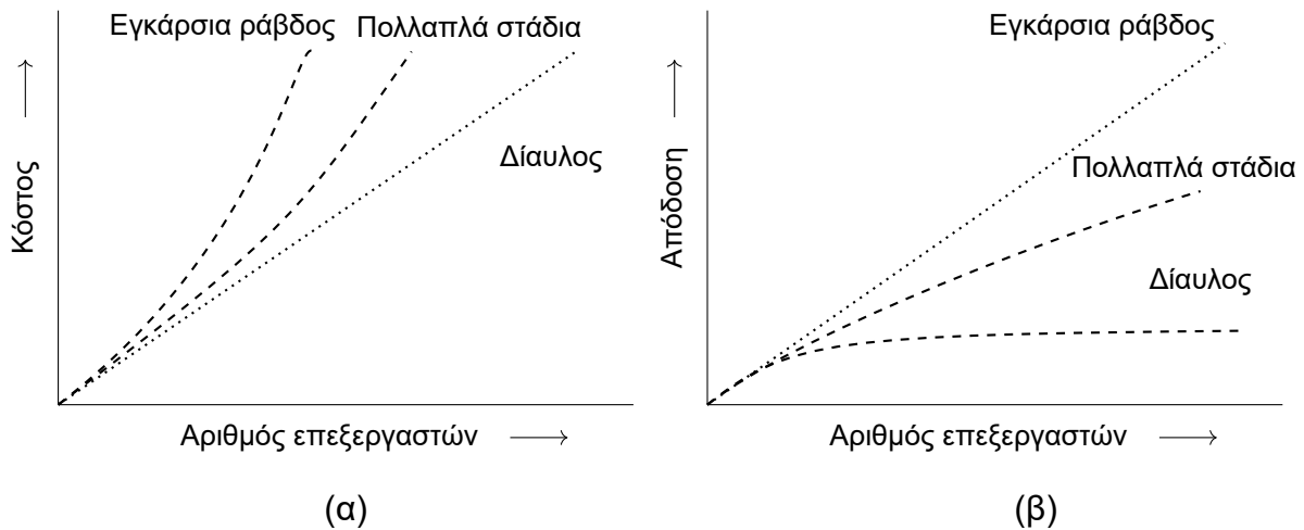
Σχήμα 9: (α) Κόστος έναντι αριθμού επεξεργασιών για δίκτυα διασύνδεσης τοπολογίας διαύλου, πολλαπλών σταδίων και συνδεδεμένα δίκτυα εγκάρσιας ράβδου (β) Απόδοση έναντι αριθμού επεξεργασιών για τα τρία δίκτυα.
