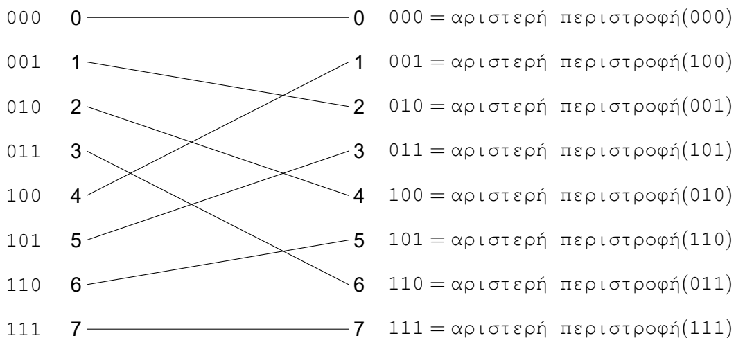
Σχήμα 10: Μια διασύνδεση τέλειου ανακατέματος για οκτώ εισόδους και εξόδους.
