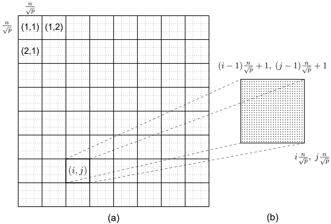
Σχήμα 44: (a) Ο πίνακας D^{(k)} διαμερισμένος με αντιστοίχιση σε μπλοκ σκακιέρας σε \sqrt{p} \times \sqrt{p} υπομπλοκ, και (b) το τετραγωνικό υπομπλοκ του D^{(k)} που ανατίθεται στον επεξεργαστή P_{i,j} .
