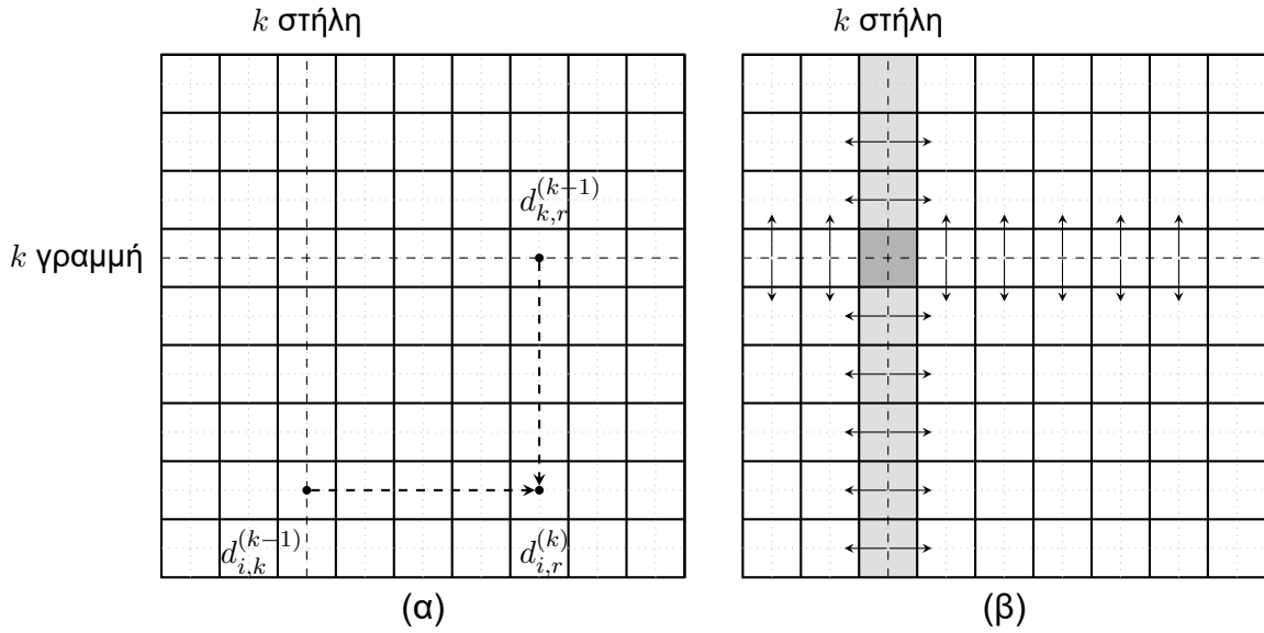
Σχήμα 45: (α) Μοτίβα επικοινωνίας που χρησιμοποιούνται στην αντιστοίχιση σε μπλοκ σκακιέρας. Κατά τον υπολογισμό του d_{i,j}^{(k)} , πληροφορίες πρέπει να αποσταλούν στον επιλεγμένο επεξεργαστή από δύο άλλους επεξεργαστές κατά μήκος της ίδιας γραμμής και στήλης. (β) Η γραμμή και η στήλη από \sqrt{p} επεξεργαστές που περιέχουν την k -οστή γραμμή και στήλη, τις αποστέλλουν κατά μήκος των στηλών και γραμμών επεξεργαστών.
