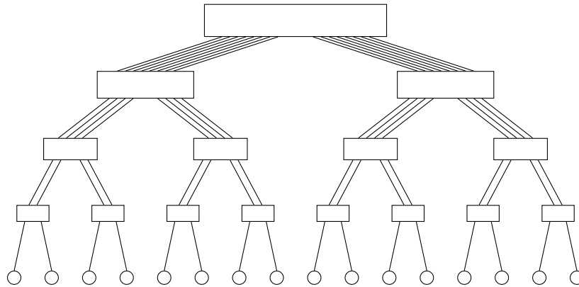
Σχήμα 18: Ένα παχύ δέντρο δικτύου με 16 επεξεργαστές.
