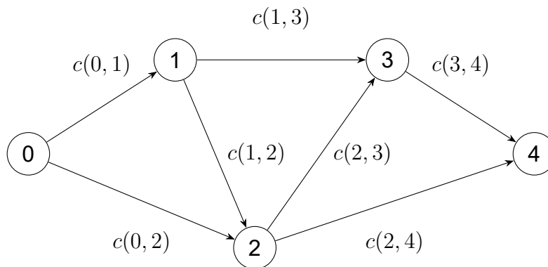
Σχήμα 58: Ένα γράφημα για το οποίο πρέπει να υπολογιστεί το συντομότερο μονοπάτι μεταξύ των κόμβων 0 και 4.
