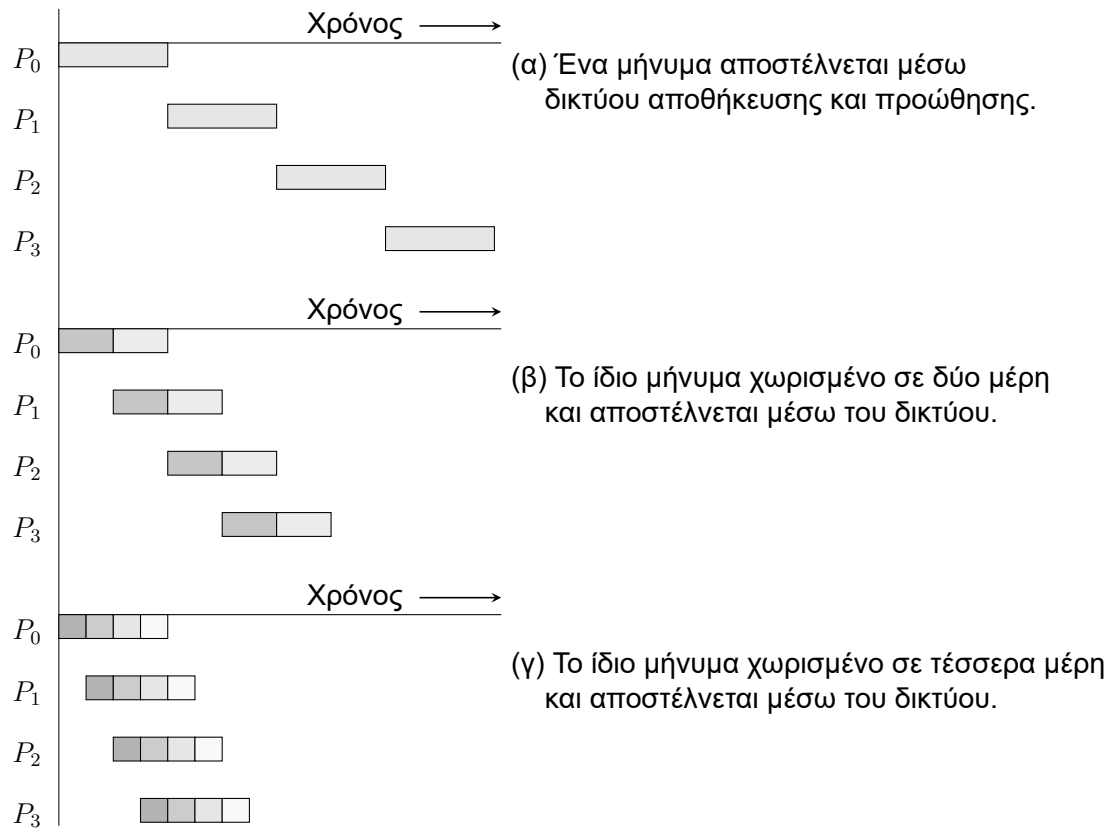
Σχήμα 26: Μεταφορά ενός μηνύματος από τον επεξεργαστή P_0 στον επεξεργαστή P_3 : (α) μέσω ενός δικτύου επικοινωνίας αποθήκευσης και προώθησης, (β) και (γ) επέκταση της ιδέας στη δρομολόγηση άμεσης προώθησης. Οι σκιασμένες περιοχές αναπαριστούν το χρονικό διάστημα κατά το οποίο το μήνυμα βρίσκεται υπό μετάδοση. Θεωρείται ότι ο χρόνος εκκίνησης που σχετίζεται με αυτή τη μεταφορά μηνύματος είναι μηδενικός.
