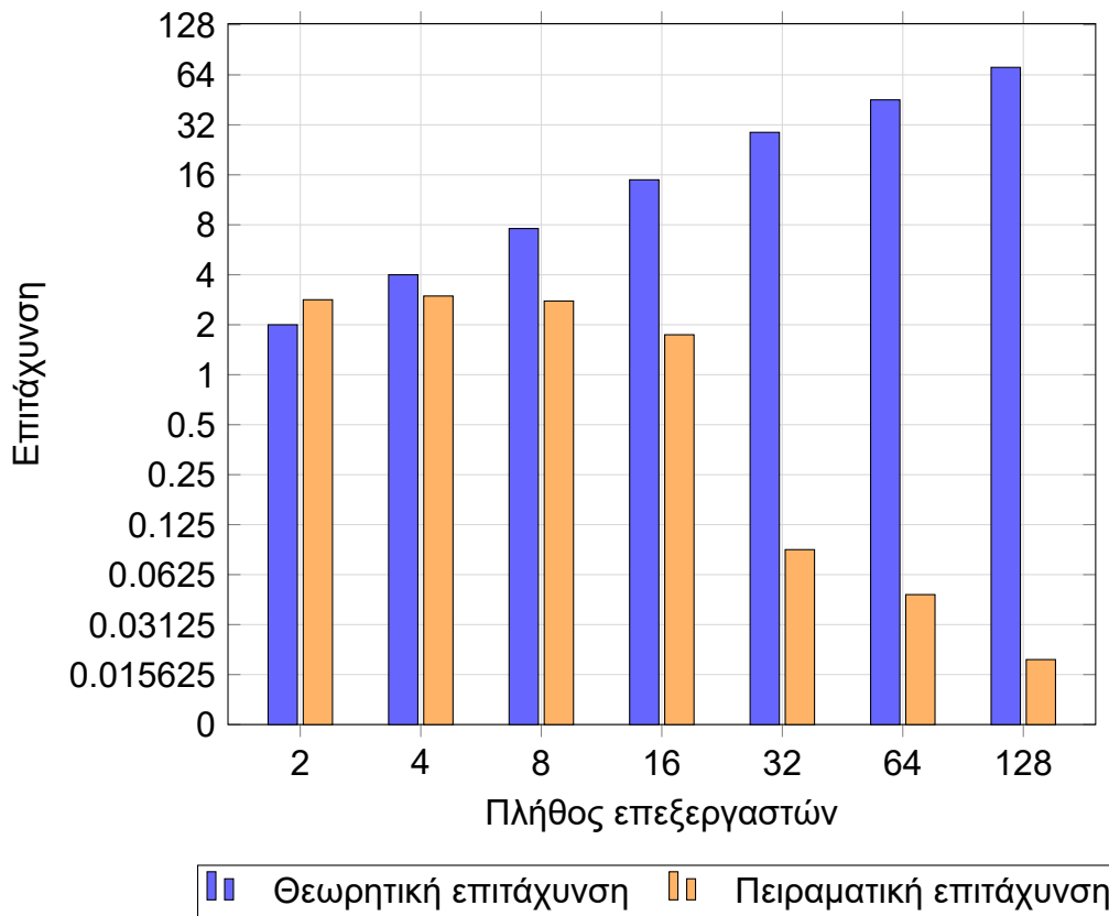
Σχήμα 41: Η σύγκριση της θεωρητικής επιτάχυνσης με την πειραματική επιτάχυνση για την υλοποίηση MPI για γράφημα 1024 κορυφών σε διαφορετικούς επεξεργαστές
