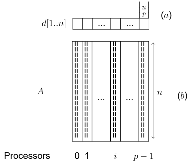
Σχήμα 37: Η διαμέριση του πίνακα απόστασης d και ο πίνακας γειτνίασης A μεταξύ p επεξεργαστών.
