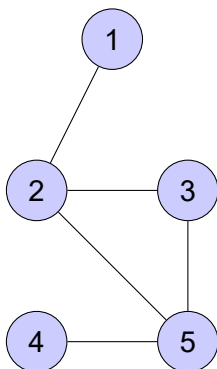
Σχήμα 33: Ένα μη κατευθυνόμενο γράφημα και η αναπαράστασή του με πίνακα γειτνίασης.
