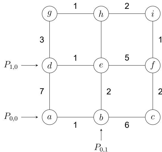
Σχήμα 52: Ένα γράφημα πλέγματος.
