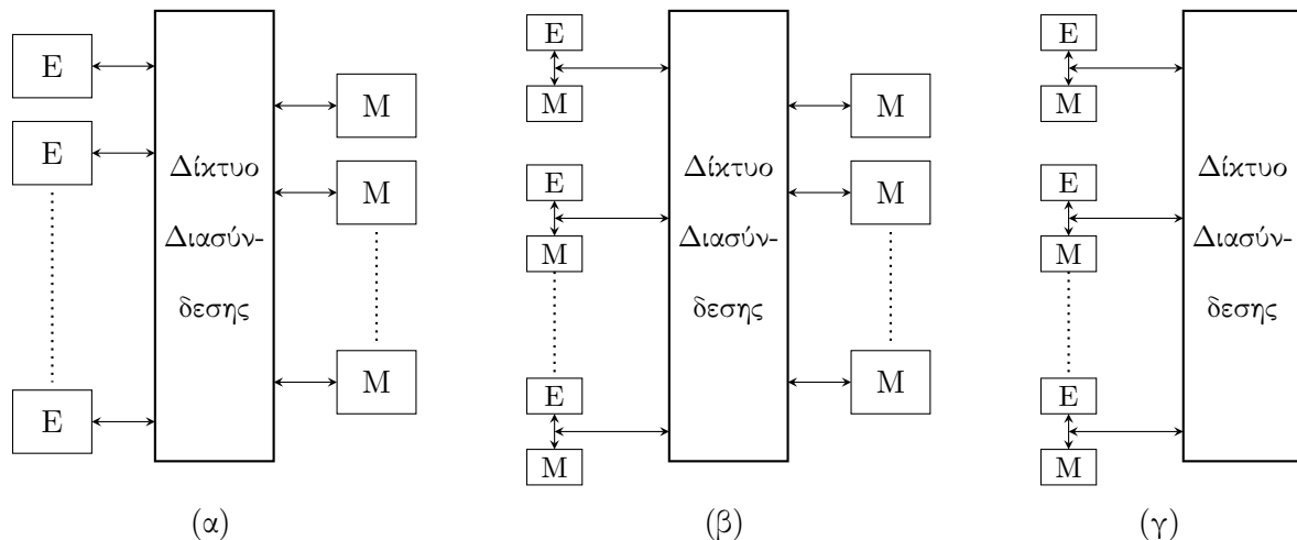
Σχήμα 5: Τυπικές αρχιτεκτονικές κοινόχρηστου χώρου διευθύνσεων: (α) Υπολογιστής κοινόχρηστου χώρου διευθύνσεων με ομοιόμορφη πρόσβαση στη μνήμη, (β) Υπολογιστής κοινόχρηστου χώρου διευθύνσεων με μη ομοιόμορφη πρόσβαση στη μνήμη, με τοπικές και καθολικές μνήμες, (γ) Υπολογιστής κοινόχρηστου χώρου διευθύνσεων με μη ομοιόμορφη πρόσβαση στη μνήμη, μόνο με τοπική μνήμη.
