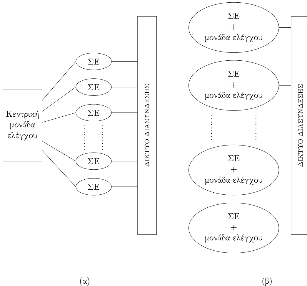
Σχήμα 2: Μία τυπική SIMD αρχιτεκτονική (α) και μία τυπική MIMD αρχιτεκτονική (β).
