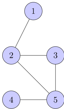
Σχήμα 2: Ένα μη κατευθυνόμενο γράφημα και η αναπαράσταση του με λίστα γειτνίασης.
