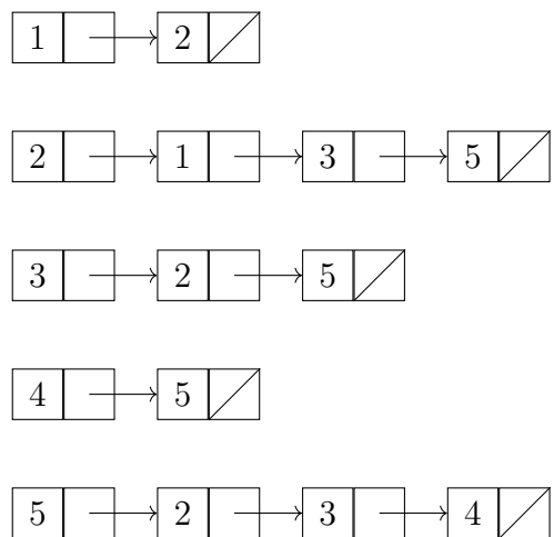
Σχήμα 3: Ένα μη κατευθυνόμενο γράφημα και η αναπαράσταση του με λίστα γειτνίασης.
