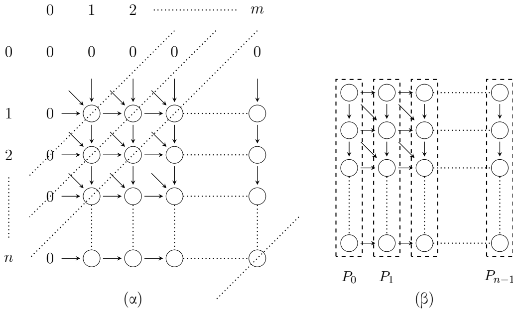
Σχήμα 31: (α) Υπολογισμός καταχωρίσεων του πίνακα F για το πρόβλημα μέγιστης κοινής υπακολουθίας. Ο υπολογισμός προχωρά κατά μήκος των διακεκομμένων διαγώνιων γραμμών. (β) Αντιστοίχιση στοιχείων του πίνακα σε επεξεργαστές.
