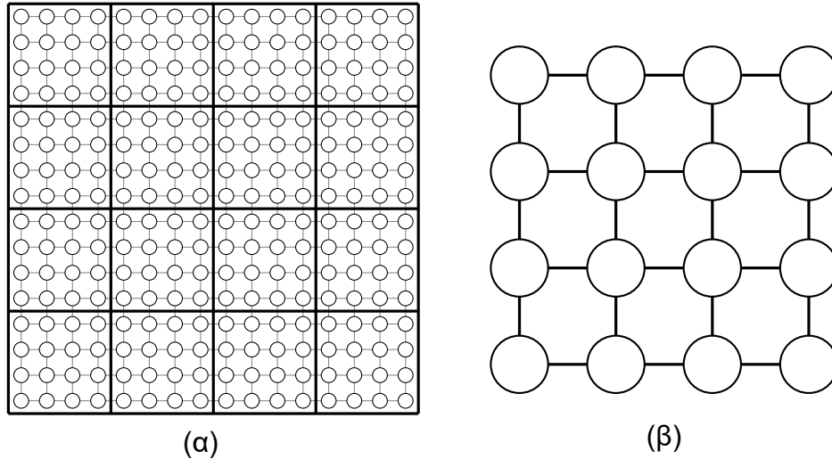
Σχήμα 54: Απεικόνιση του γραφήματος πλέγματος (α) σε ένα πλέγμα (β) χρησιμοποιώντας την απεικόνιση μπλοκ σκακιάρας. Σε αυτό το παράδειγμα, n = 16 και \sqrt{p} = 4 . Οι σκιασμένες κορυφές απεικονίζονται στον σκιασμένο επεξεργαστή.
