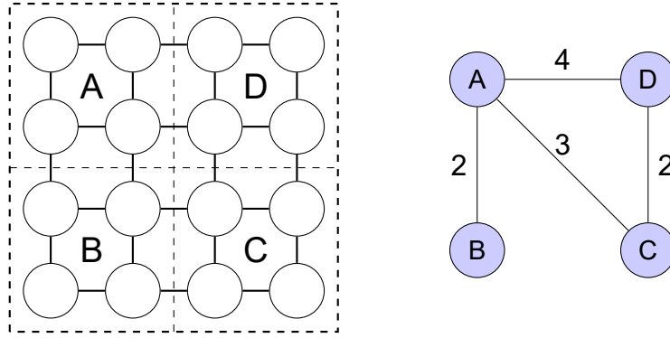
Σχήμα 43: Διαμέριση ενός πλέγματος \sqrt{p} \times \sqrt{p} σε n υποπλέγματα, καθένα με μέγεθος \sqrt{p/n} \times \sqrt{p/n} . Στο παράδειγμα αυτό, p = 16 και n = 4 . Κάθε ένα από τα πλέγματα μεγέθους \sqrt{p/n} \times \sqrt{p/n} = 2 \times 2 επιλύει το πρόβλημα των συντομότερων διαδρομών μονής πηγής για μια δοσμένη κορυφή πηγής. Στο παράδειγμα αυτό, κάθε υποπλέγμα επισημαίνεται από την κορυφή πηγής του αντίστοιχου αλγορίθμου μονής πηγής.
