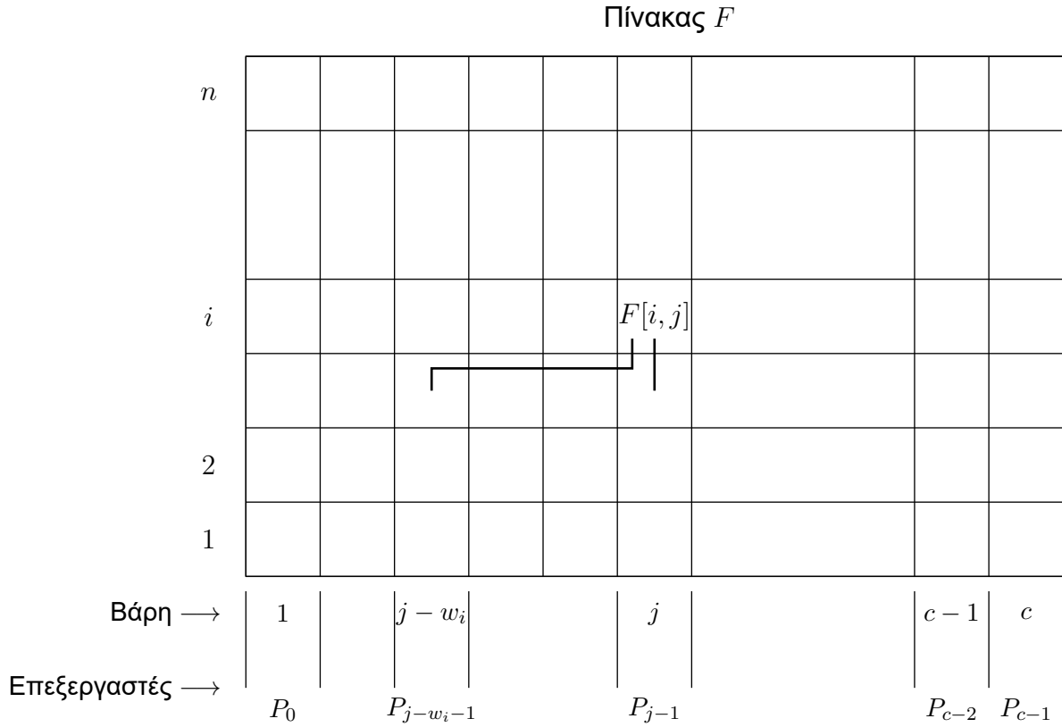
Σχήμα 61: Υπολογισμός καταχωρίσεων του πίνακα F για το πρόβλημα σακιδίου 0/1. Ο υπολογισμός της καταχώρισης F[i, j] απαιτεί επικοινωνία με επεξεργαστές που περιέχουν τις καταχωρίσεις F[i-1, j] και F[i-1, j-w_i] .
