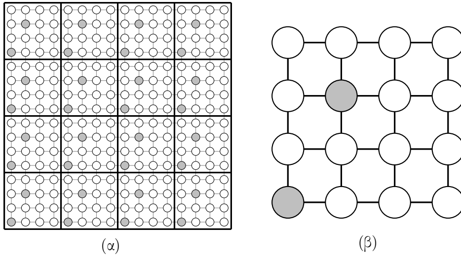
Σχήμα 24: Απεικόνιση του γραφήματος πλέγματος (α) σε ένα πλέγμα (β) χρησιμοποιώντας την απεικόνιση μπλοκ σκακιέρας. Σε αυτό το παράδειγμα, n = 16 και \sqrt{p} = 4 . Οι σκιασμένες κορυφές απεικονίζονται στους αντίστοιχους σκιασμένους επεξεργαστές πλέγματος.
