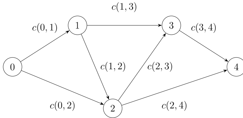
Σχήμα 55: Ένα γράφημα για το οποίο πρέπει να υπολογιστεί το συντομότερο μονοπάτι μεταξύ των κόμβων 0 και 4.
