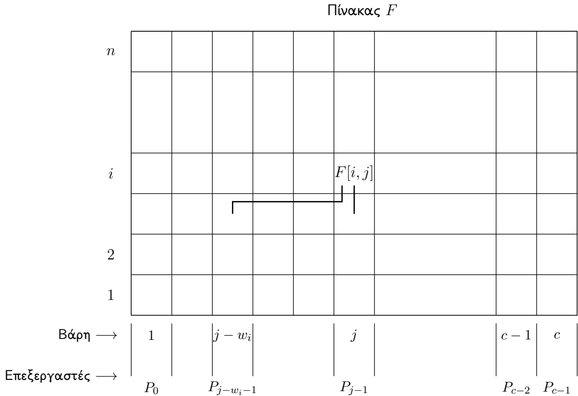
Σχήμα 61: Υπολογισμός καταχωρίσεων του πίνακα F για το πρόβλημα σακιδίου 0/1. Ο υπολογισμός της καταχώρισης F[i, j] απαιτεί επικοινωνία με επεξεργαστές που περιέχουν τις καταχωρίσεις F[i - 1, j] και F[i - 1, j - w_i] .
