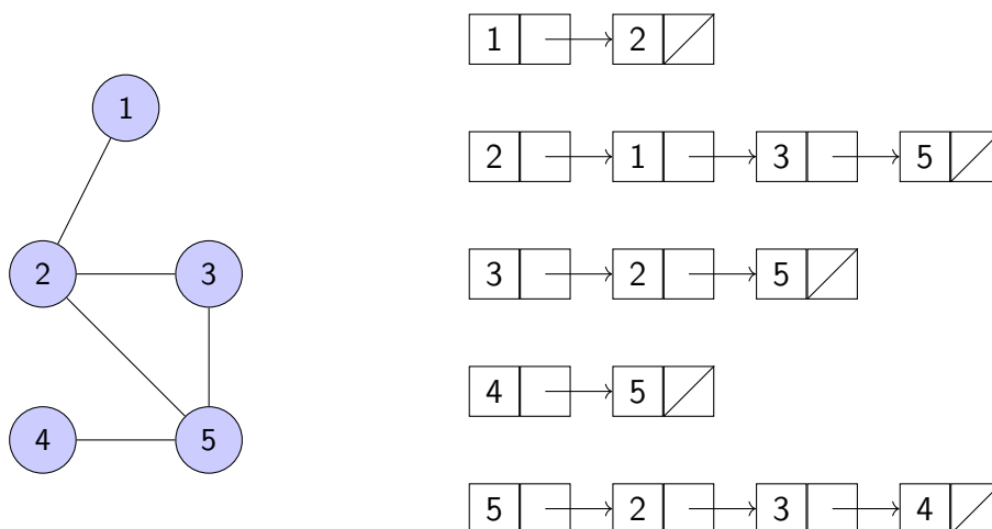
Σχήμα 34: Ένα μη κατευθυνόμενο γράφημα και η αναπαράστασή του με λίστα γειτνίασης.
