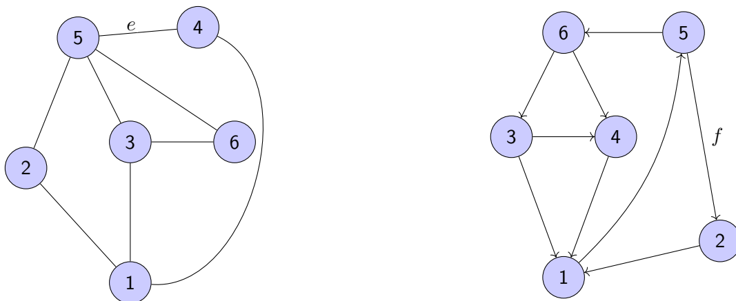
Σχήμα 32: (α) Ένα μη κατευθυνόμενο γράφημα και (β) ένα κατευθυνόμενο γράφημα.
