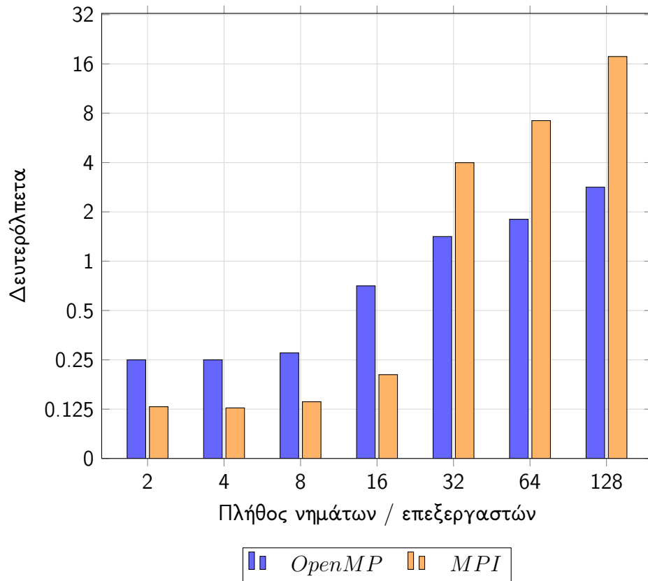
Σχήμα 39: Διαφορετικά νήματα/επεξεργαστές για την υλοποίηση OpenMP και MPI σε γράφημα με 1024 κορυφές
