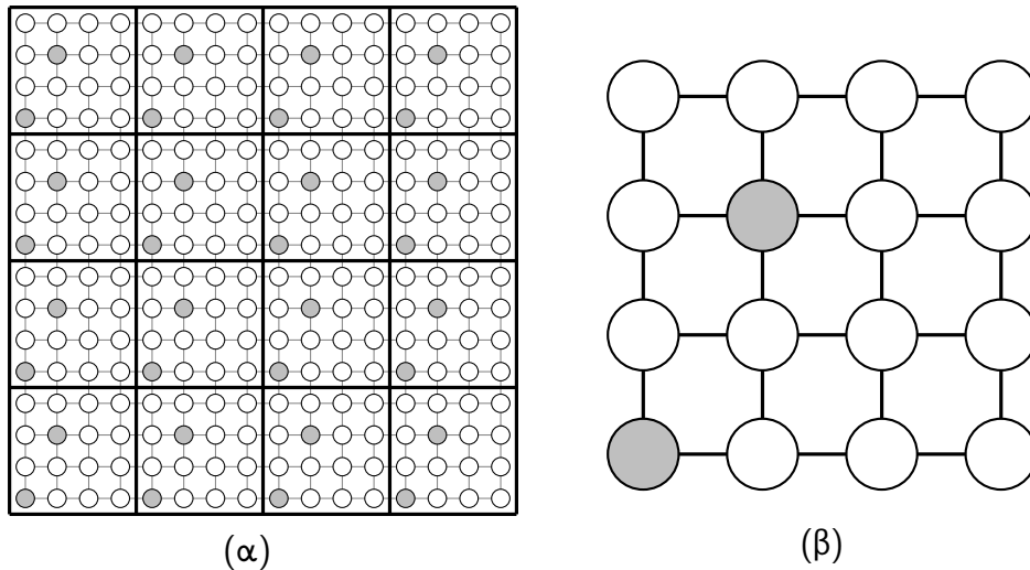
Σχήμα 55: Απεικόνιση του γραφήματος πλέγματος (α) σε ένα πλέγμα (β) χρησιμοποιώντας την κυκλική απεικόνιση σκακιέρας. Σε αυτό το παράδειγμα, n = 16 και \sqrt{p} = 4 . Οι σκιασμένες κορυφές απεικονίζονται στους αντίστοιχους σκιασμένους επεξεργαστές πλέγματος.
