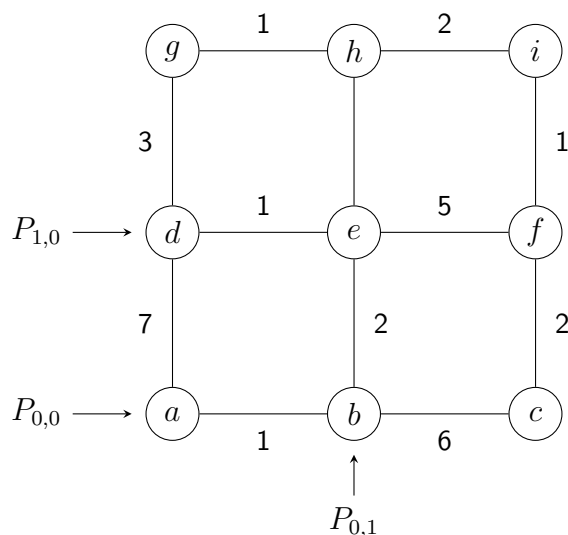
Σχήμα 52: Ένα γράφημα πλέγματος.
