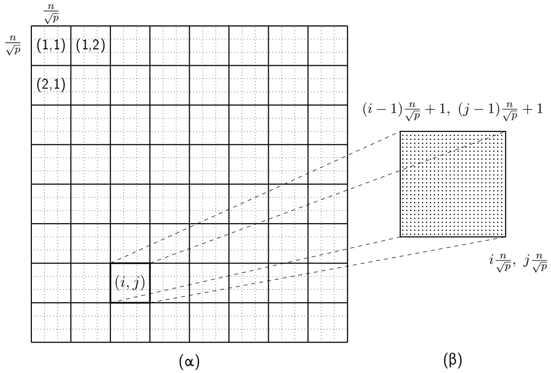
Σχήμα 44: (α) Ο πίνακας D^{(k)} διαμερισμένος με αντιστοίχιση σε μπλοκ σκακιέρας σε \sqrt{p} \times \sqrt{p} υπομπλοκ, και (β) το τετραγωνικό υπομπλοκ του D^{(k)} που ανατίθεται στον επεξεργαστή P_{i,j} .
