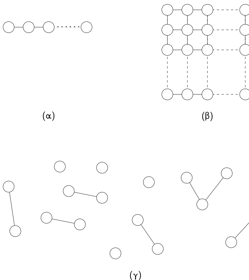
Σχήμα 50: Παραδείγματα αραιών γραφημάτων: (α) ένα γραμμικό γράφημα, στον οποίο κάθε κορυφή έχει δύο προσπίπτουσες ακμές, (β) ένα γράφημα πλέγματος, στον οποίο κάθε κορυφή έχει τέσσερις γειτονικές κορυφές και (γ) τυχαίο αραιό γράφημα.
