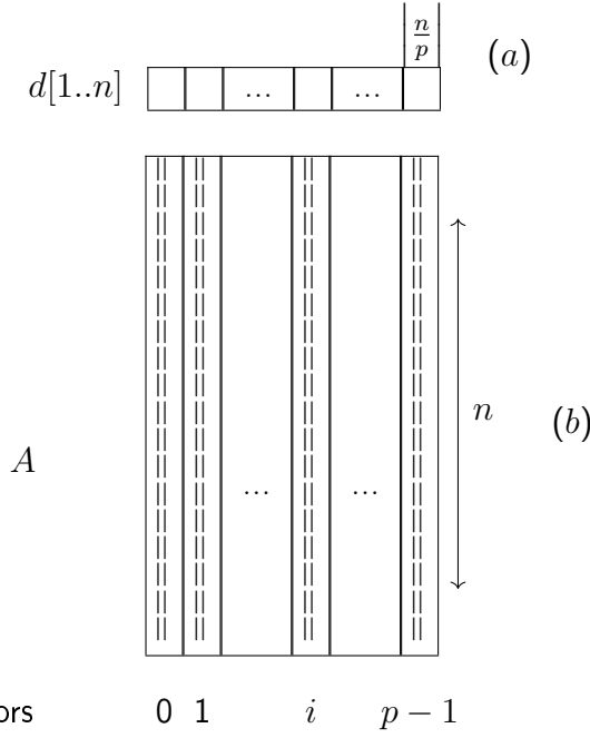
Σχήμα 37: Η διαμέριση του πίνακα απόστασης d και ο πίνακας γειτνίασης A μεταξύ p επεξεργαστών.
