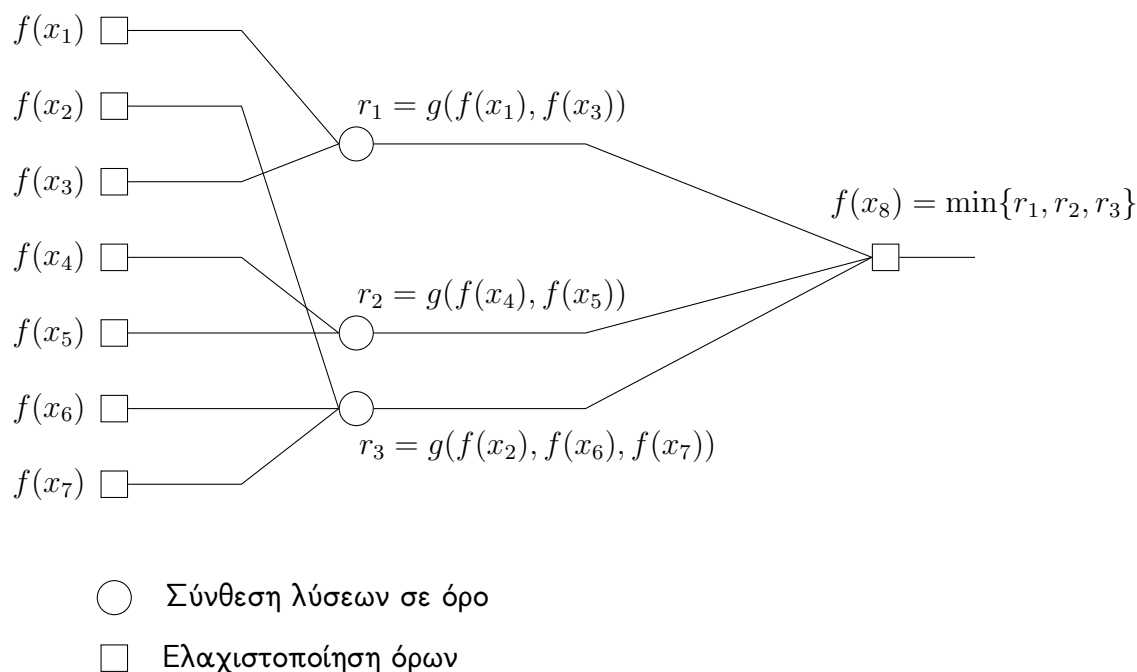
Σχήμα 59: Ο υπολογισμός και η σύνθεση λύσεων υποπροβλημάτων για την επίλυση του προβλήματος f(x_8) .
