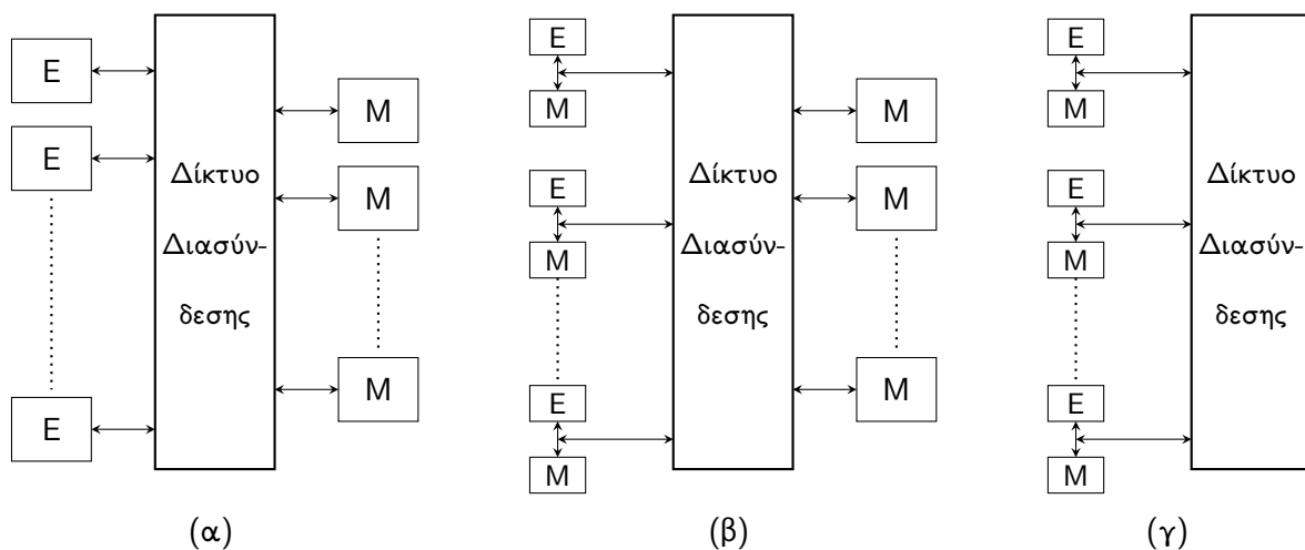
Σχήμα 5: Τυπικές αρχιτεκτονικές κοινόχρηστου χώρου διευθύνσεων: (α) Υπολογιστής κοινόχρηστου χώρου διευθύνσεων με ομοιόμορφη πρόσβαση στη μνήμη, (β) Υπολογιστής κοινόχρηστου χώρου διευθύνσεων με μη ομοιόμορφη πρόσβαση στη μνήμη, με τοπικές και καθολικές μνήμες, (γ) Υπολογιστής κοινόχρηστου χώρου διευθύνσεων με μη ομοιόμορφη πρόσβαση στη μνήμη, μόνο με τοπική μνήμη.
