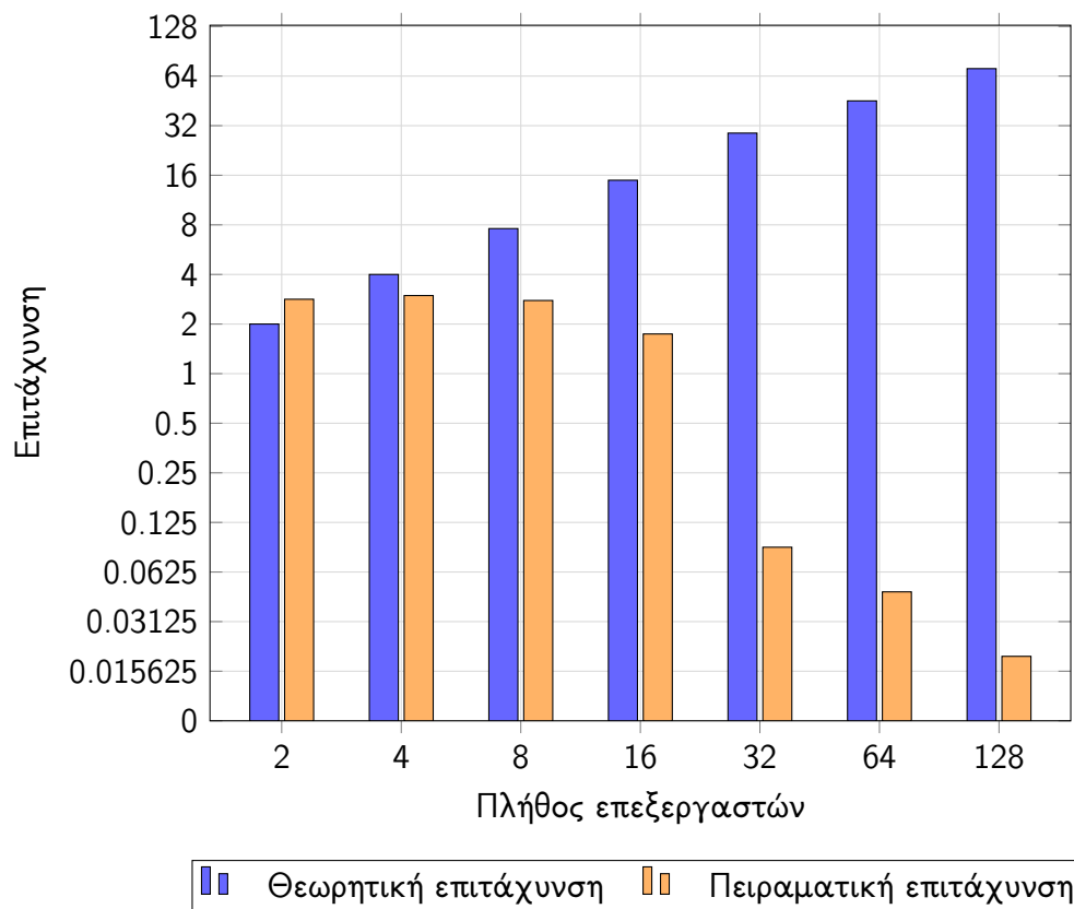
Σχήμα 41: Η σύγκριση της θεωρητικής επιτάχυνσης με την πειραματική επιτάχυνση για την υλοποίηση MPI για γράφημα 1024 κορυφών σε διαφορετικούς επεξεργαστές
