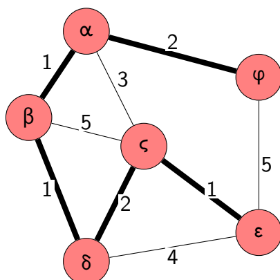
(δ) Τελικό ελάχιστο δέντρο επικάλυψης
