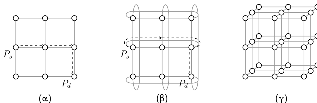
Σχήμα 16: (α) Ένα διδιάστατο πλέγμα με παράδειγμα δρομολόγησης ενός μηνύματος από τον επεξεργαστή P_s στον επεξεργαστή P_d . (β) Ένα διδιάστατο πλέγμα με σύνδεση αναδίπλωσης με παράδειγμα δρομολόγησης ενός μηνύματος από τον επεξεργαστή P_s στον επεξεργαστή P_d . (γ) Ένα τριδιάστατο πλέγμα.
