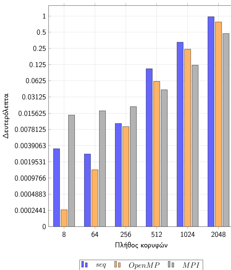
Σχήμα 38: Ο καλύτερος χρόνος εκτέλεσης για κάθε υλοποίηση σε διαφορετικά σύνολα δεδομένων
