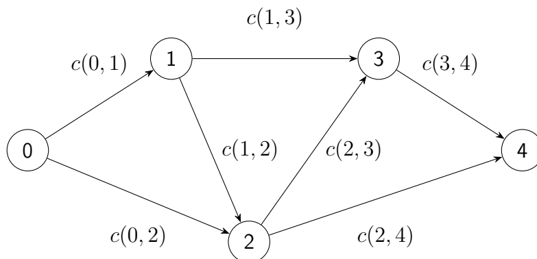
Σχήμα 58: Ένα γράφημα για το οποίο πρέπει να υπολογιστεί το συντομότερο μονοπάτι μεταξύ των κόμβων 0 και 4.
