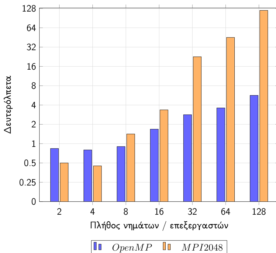
Σχήμα 40: Διαφορετικά νήματα/επεξεργαστές για την υλοποίηση OpenMP και MPI σε γράφημα με 2048 κορυφές
