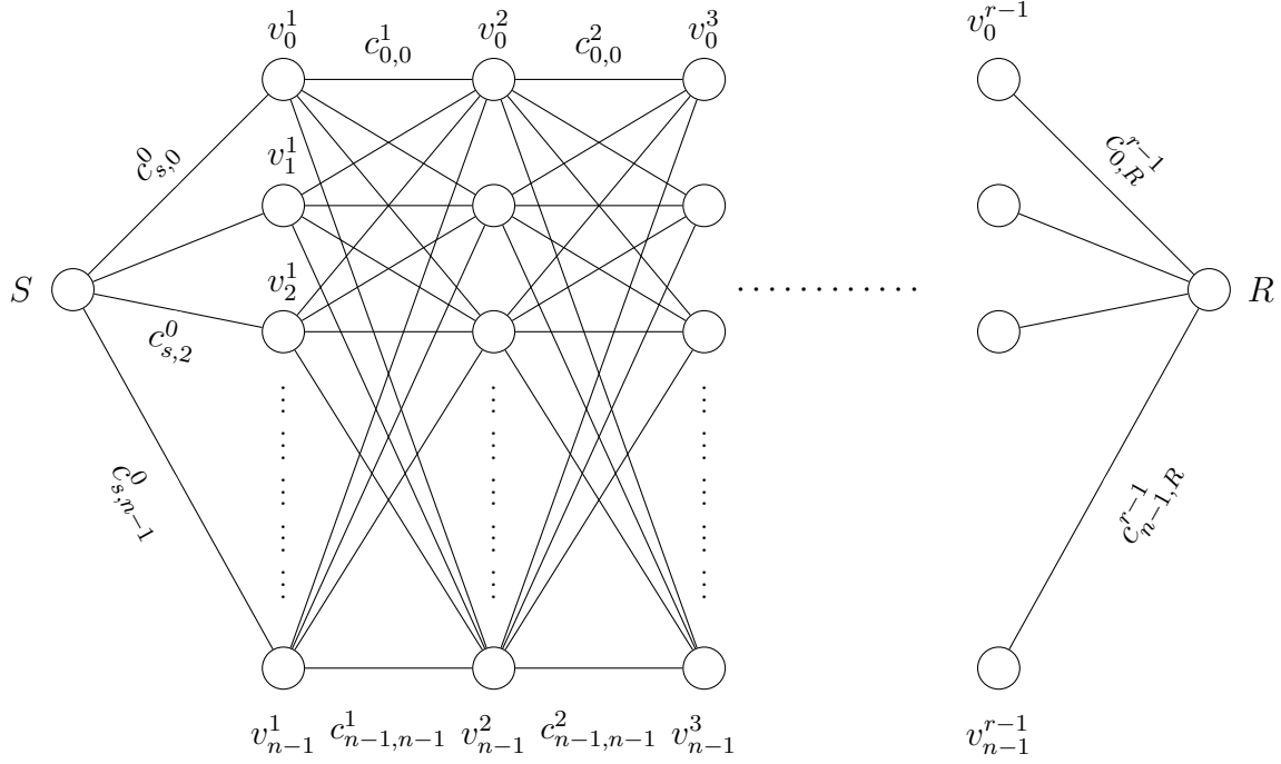
Σχήμα 60: Ένα παράδειγμα σειριακής μοναδικής υλοποίησης ΔΠ για την εύρεση του συντομότερου μονοπατιού σε ένα γράφημα του οποίου οι κόμβοι μπορούν να οργανωθούν σε επίπεδα.
