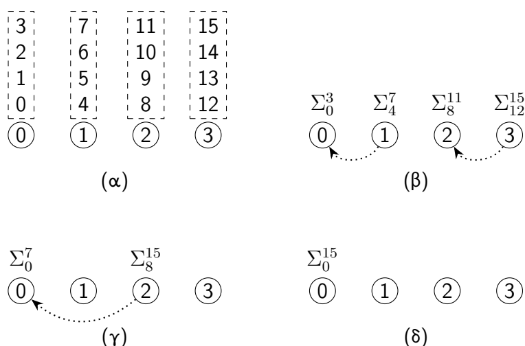
Σχήμα 30: Ένας βέλτιστος ως προς το κόστος τρόπος υπολογισμού του αθροίσματος 16 αριθμών σε έναν υπερκύβο τεσσάρων επεξεργαστών.
