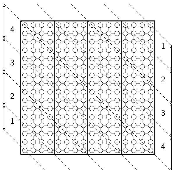
Σχήμα 57: Ο αριθμός των απασχολημένων επεξεργαστών αυξάνεται καθώς το κύμα διαδίδεται μέσα από το γράφημα πλέγματος.
