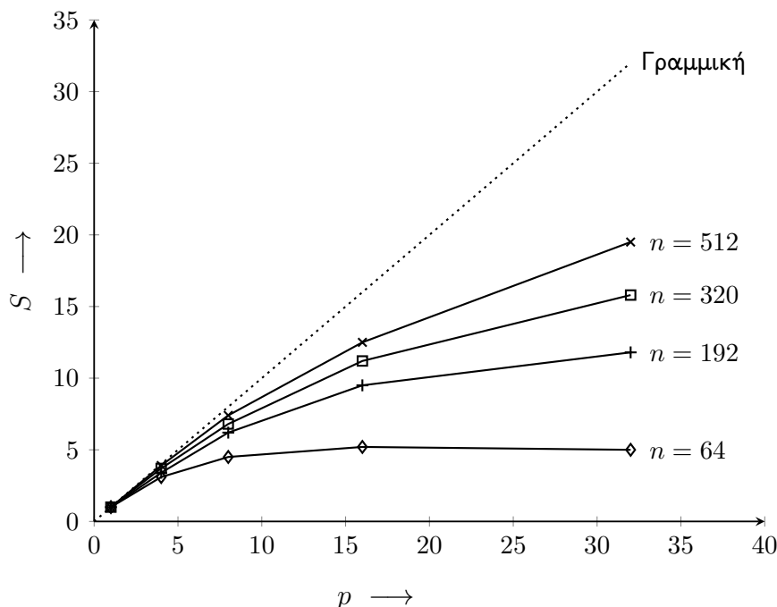
Σχήμα 31: Επιτάχυνση εναντίον του αριθμού των επεξεργαστών για την άθροιση μιας λίστας αριθμών σε έναν υπερκύβο.
