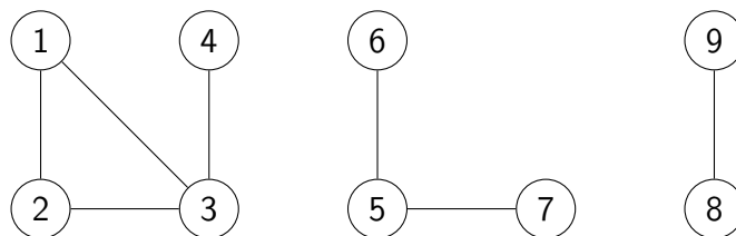
Σχήμα 47: Ένα γράφημα με τρεις συνεκτικές συνιστώσες: \{1, 2, 3, 4\} , \{5, 6, 7\} , και \{8, 9\} .
