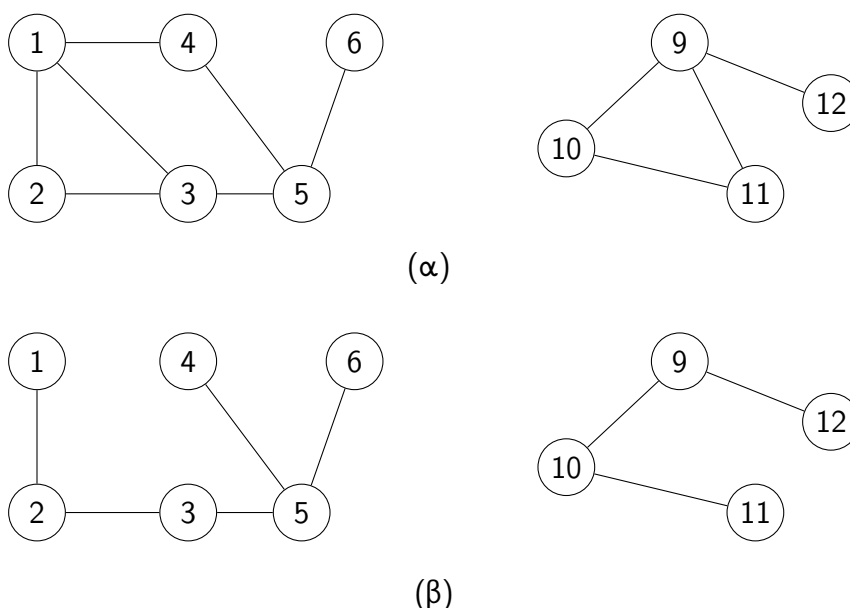
Σχήμα 48: Το μέρος (β) είναι ένα δάσος πρώτα κατά βάθος που προκύπτει από διάσχιση πρώτα κατά βάθος του γραφήματος στο μέρος (α). Κάθε ένα από αυτά τα δέντρα είναι μια συνεκτική συνιστώσα του γραφήματος στο μέρος (α).
