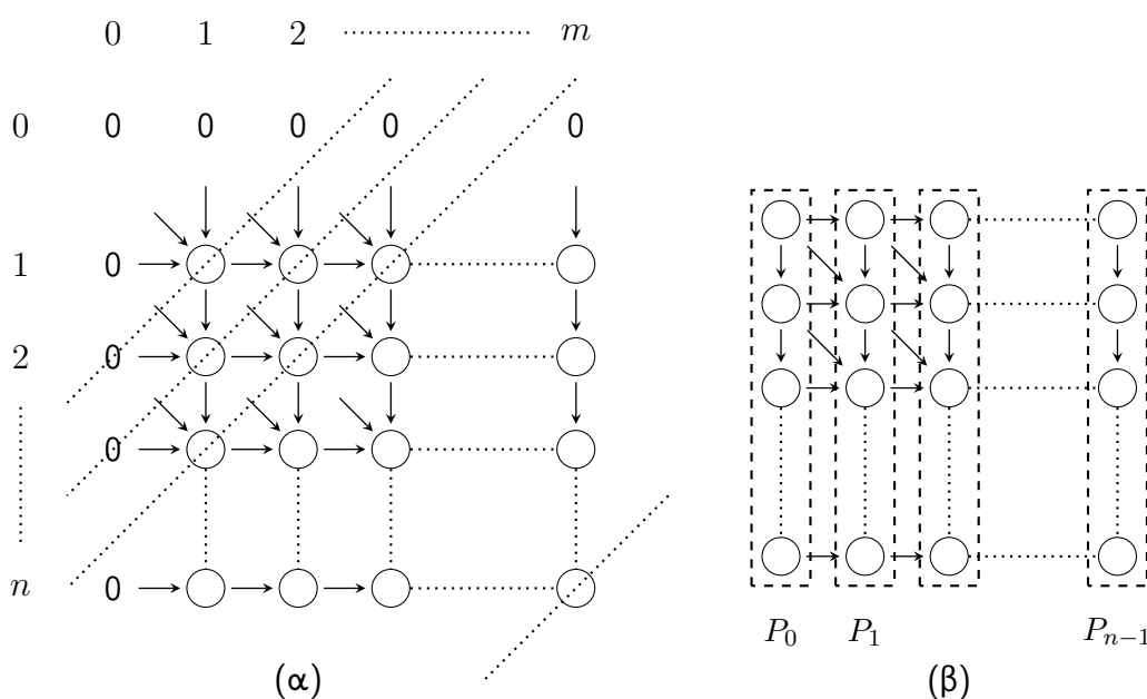
Σχήμα 62: (α) Υπολογισμός καταχωρίσεων του πίνακα F για το πρόβλημα μέγιστης κοινής υπακολουθίας. Ο υπολογισμός προχωρά κατά μήκος των διακεκομμένων διαγώνιων γραμμών. (β) Αντιστοίχιση στοιχείων του πίνακα σε επεξεργαστές.
