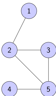
Σχήμα 33: Ένα μη κατευθυνόμενο γράφημα και η αναπαράστασή του με πίνακα γειτνιάσεων.
