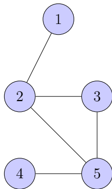
Σχήμα 33: Ένα μη κατευθυνόμενο γράφημα και η αναπαράσταση του με πίνακα γειτνίασης.
