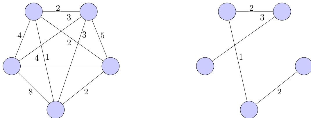
Σχήμα 9: Ένα μη κατευθυνόμενο γράφημα και το ελάχιστο δέντρο επικάλυψης του.
