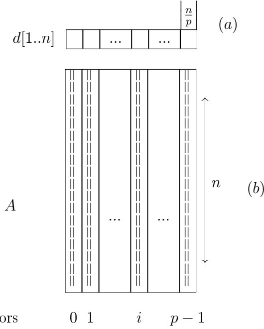
Σχήμα 11: Η διαμέριση του πίνακα απόστασης d και ο πίνακας γειτνίασης A μεταξύ p επεξεργαστών.
