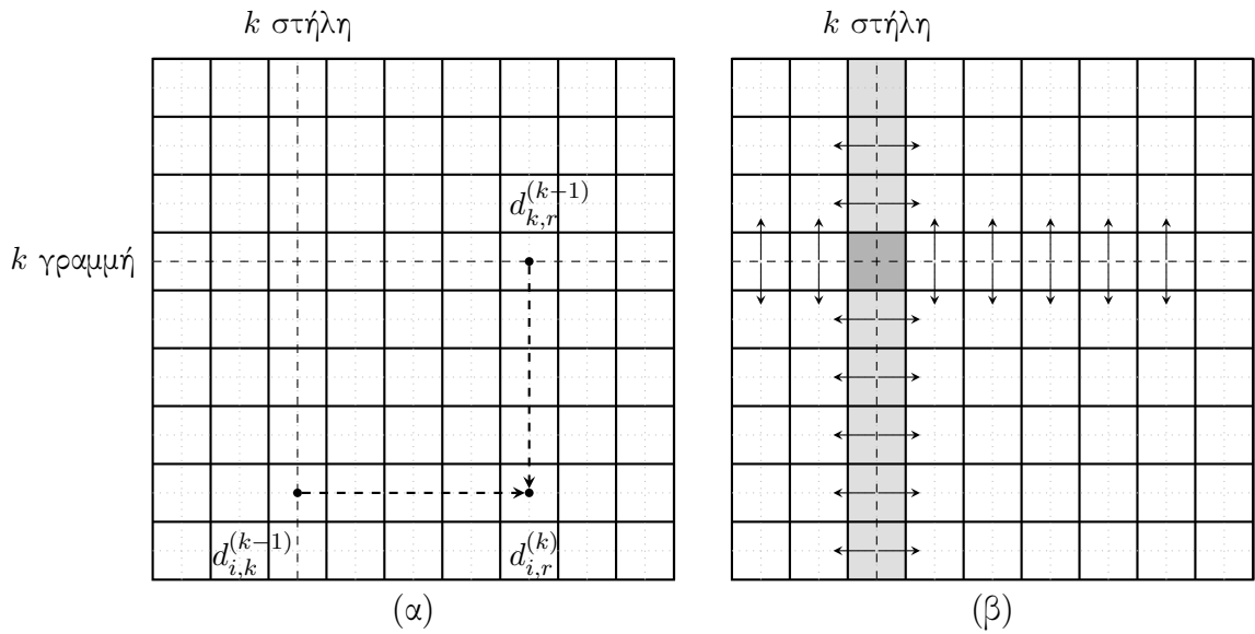
Σχήμα 19: (α) Μοτίβα επικοινωνίας που χρησιμοποιούνται στην αντιστοίχιση σε μπλοκ σκακιέρας. Κατά τον υπολογισμό του d_{i,j}^{(k)} , πληροφορίες πρέπει να αποσταλούν στον επιλεγμένο επεξεργαστή από δύο άλλους επεξεργαστές κατά μήκος της ίδιας γραμμής και στήλης. (β) Η γραμμή και η στήλη από \sqrt{p} επεξεργαστές που περιέχουν την k -οστή γραμμή και στήλη, τις αποστέλλουν κατά μήκος των στηλών και γραμμών επεξεργαστών.
