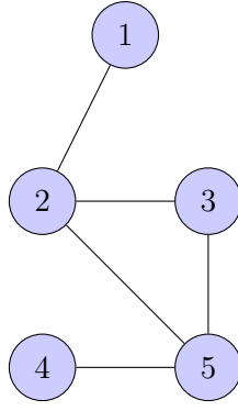
Σχήμα 7: Ένα μη κατευθυνόμενο γράφημα και η αναπαράστασή του με πίνακα γειτνίασης.
