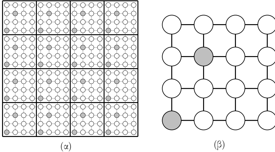
Σχήμα 29: Απεικόνιση του γραφήματος πλέγματος (α) σε ένα πλέγμα (β) χρησιμοποιώντας την κυκλική απεικόνιση σκακιέρας. Σε αυτό το παράδειγμα, n = 16 και \sqrt{p} = 4 . Οι σκιασμένες κορυφές απεικονίζονται στους αντίστοιχους σκιασμένους επεξεργαστές πλέγματος.
