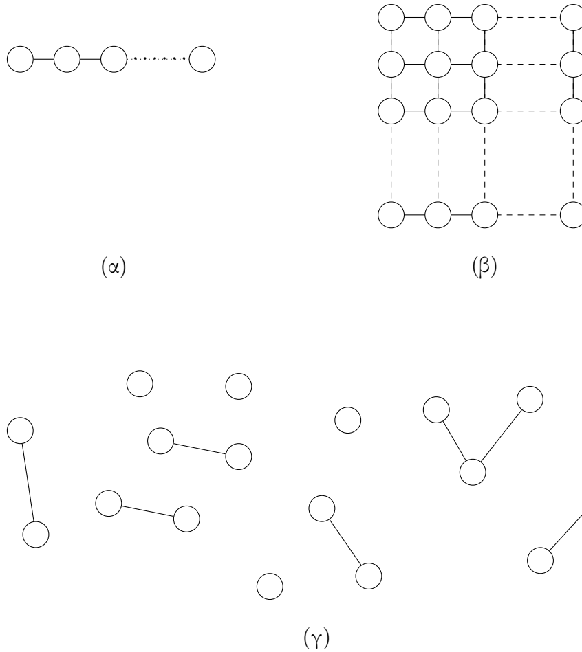
Σχήμα 24: Παραδείγματα αραιών γραφημάτων: (α) ένα γραμμικό γράφημα, στον οποίο κάθε κορυφή έχει δύο προσπίπτουσες ακμές, (β) ένα γράφημα πλέγματος, στον οποίο κάθε κορυφή έχει τέσσερις γειτονικές κορυφές και (γ) τυχαίο αραιό γράφημα.
