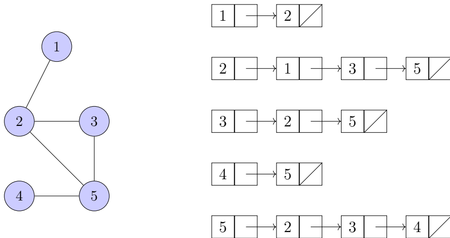
Σχήμα 8: Ένα μη κατευθυνόμενο γράφημα και η αναπαράστασή του με λίστα γειτνίασης.
