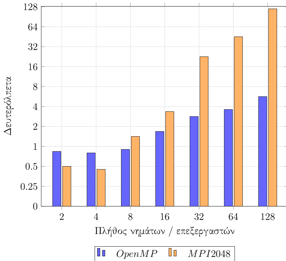
Σχήμα 11: Διαφορετικά νήματα/επεξεργαστές για την υλοποίηση OpenMP και MPI σε γράφημα με 2048 κορυφές
