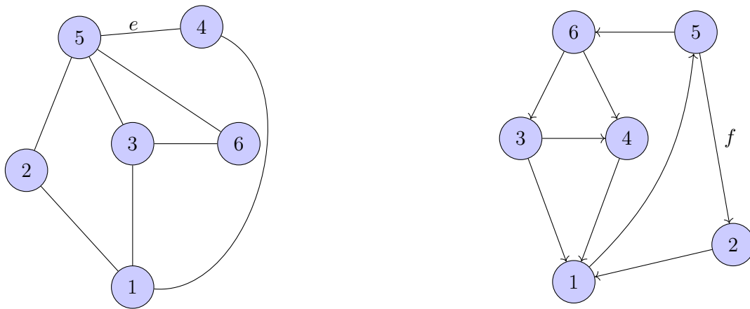
Σχήμα 3: (α) Ένα μη κατευθυνόμενο γράφημα και (β) ένα κατευθυνόμενο γράφημα.
