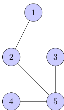
Σχήμα 4: Ένα μη κατευθυνόμενο γράφημα και η αναπαράσταση του με λίστα γειτνίασης.
