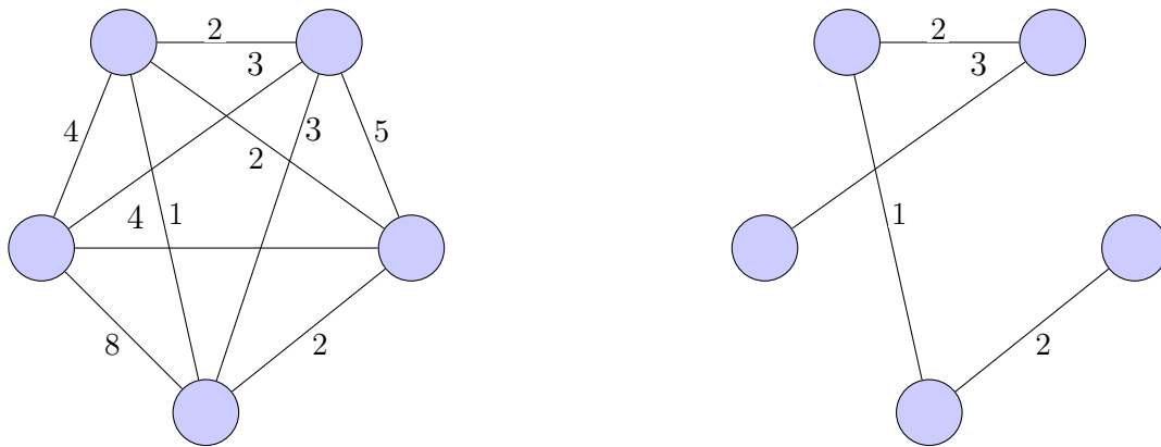
Σχήμα 6: Ένα μη κατευθυνόμενο γράφημα και το ελάχιστο δέντρο επικάλυψης του.
