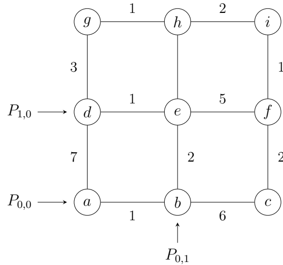
Σχήμα 23: Ένα γράφημα πλέγματος.
