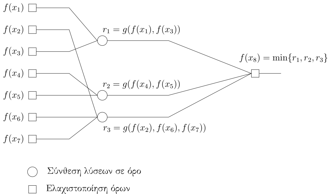
Σχήμα 29: Ο υπολογισμός και η σύνθεση λύσεων υποπροβλημάτων για την επίλυση του προβλήματος f(x_8) .
