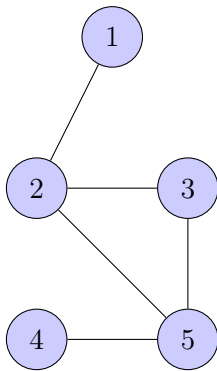
Σχήμα 3: Ένα μη κατευθυνόμενο γράφημα και η αναπαράσταση του με λίστα γειτνίασης.
