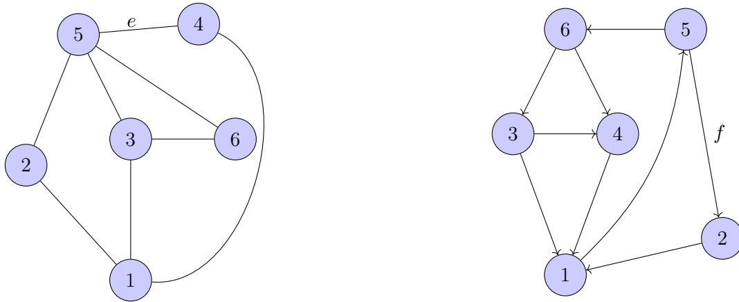
Σχήμα 2: (α) Ένα μη κατευθυνόμενο γράφημα και (β) ένα κατευθυνόμενο γράφημα.
