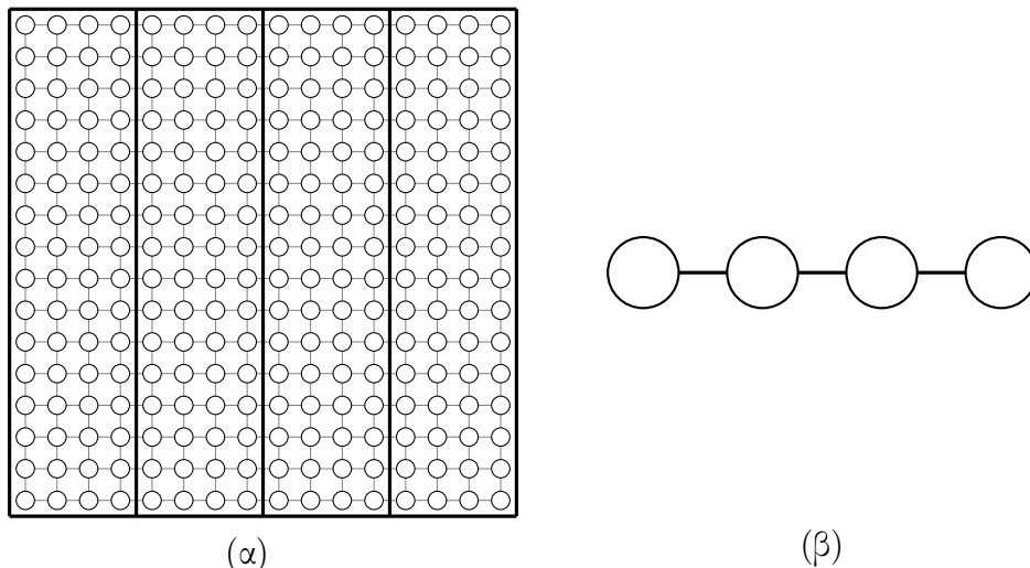
Σχήμα 26: Απεικόνιση του γραφήματος πλέγματος (α) σε ένα γραμμικό πίνακα από επεξεργαστές (β). Σε αυτό το παράδειγμα, n = 16 και \sqrt{p} = 4 . Οι σκιασμένες κορυφές απεικονίζονται στον σκιασμένο επεξεργαστή.
