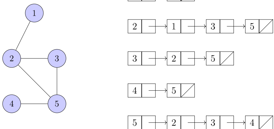
Σχήμα 4: Ένα μη κατευθυνόμενο γράφημα και η αναπαράστασή του με λίστα γειτνίασης.
