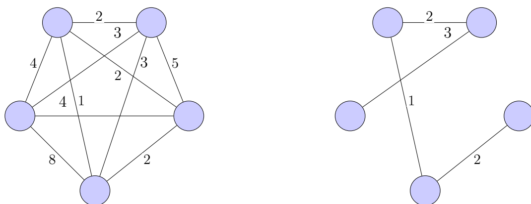
Σχήμα 5: Ένα μη κατευθυνόμενο γράφημα και το ελάχιστο δέντρο επικάλυψής του.
