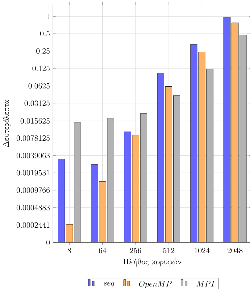
Σχήμα 31: Ο καλύτερος χρόνος εκτέλεσης για κάθε υλοποίηση σε διαφορετικά σύνολα δεδομένων
