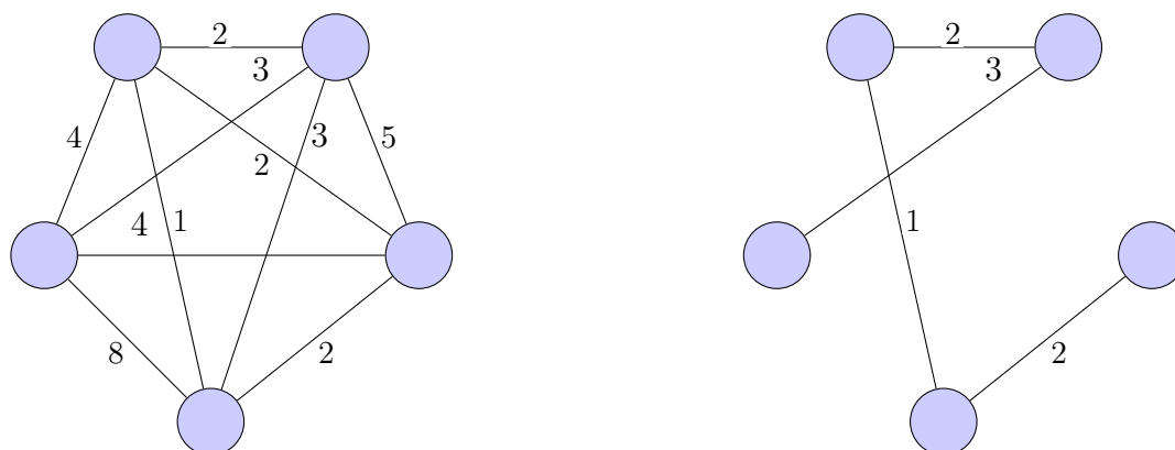
Σχήμα 28: Ένα μη κατευθυνόμενο γράφημα και το ελάχιστο δέντρο επικάλυψης του.
