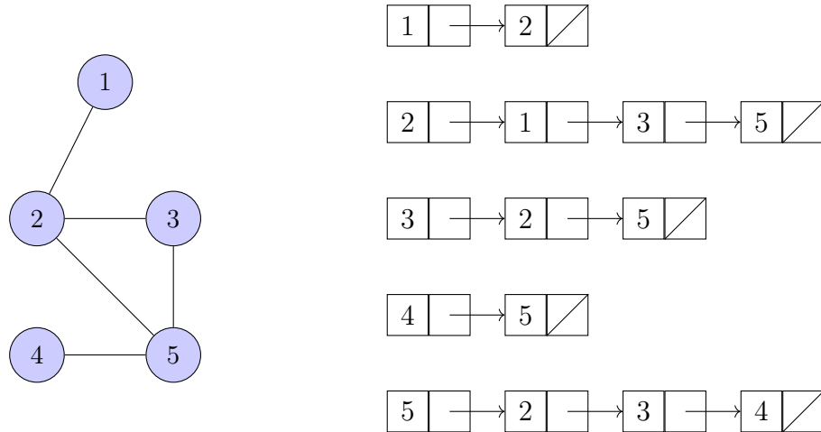
Σχήμα 27: Ένα μη κατευθυνόμενο γράφημα και η αναπαράστασή του με λίστα γειτνίασης.
