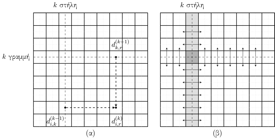
Σχήμα 38: (α) Μοτίβα επικοινωνίας που χρησιμοποιούνται στην αντιστοίχιση σε μπλοκ σκακιέρας. Κατά τον υπολογισμό του d_{i,j}^{(k)} , πληροφορίες πρέπει να αποσταλούν στον επιλεγμένο επεξεργαστή από δύο άλλους επεξεργαστές κατά μήκος της ίδιας γραμμής και στήλης. (β) Η γραμμή και η στήλη από \sqrt{p} επεξεργαστές που περιέχουν την k -οστή γραμμή και στήλη, τις αποστέλλουν κατά μήκος των στηλών και γραμμών επεξεργαστών.
