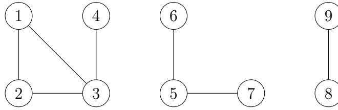
Σχήμα 40: Ένα γράφημα με τρεις συνεκτικές συνιστώσες: \{1, 2, 3, 4\} , \{5, 6, 7\} , και \{8, 9\} .
