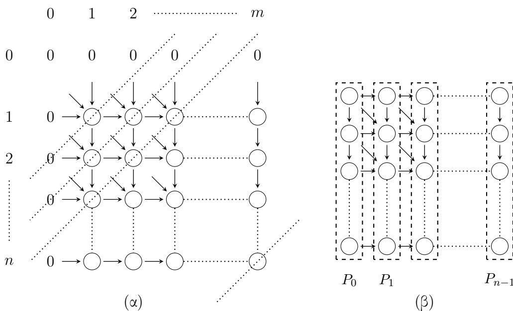
Σχήμα 55: (α) Υπολογισμός καταχωρίσεων του πίνακα F για το πρόβλημα μέγιστης κοινής υποακολουθίας. Ο υπολογισμός προχωρά κατά μήκος των διακεκομμένων διαγώνιων γραμμών. (β) Αντιστοίχιση στοιχείων του πίνακα σε επεξεργαστές.
