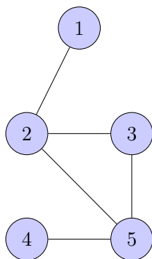
Σχήμα 26: Ένα μη κατευθυνόμενο γράφημα και η αναπαράσταση του με πίνακα γειτνίασης.
