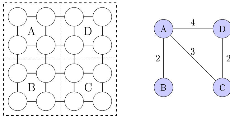
Σχήμα 12: Ένα παράδειγμα του αλγορίθμου για τις συντομότερες διαδρομές μεταξύ όλων των ζευγών.
