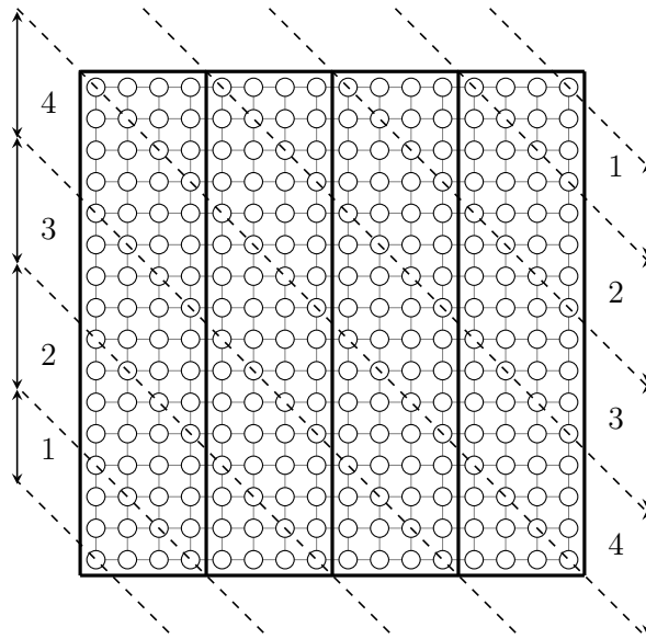
Σχήμα 32: Ο αριθμός των απασχολημένων επεξεργαστών αυξάνεται καθώς το κύμα διαδίδεται μέσα από το γράφημα πλέγματος.
