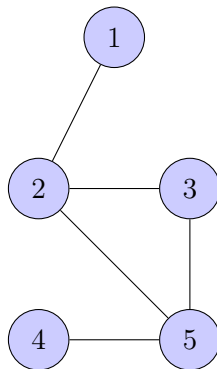
Σχήμα 8: Ένα μη κατευθυνόμενο γράφημα και η αναπαράσταση του με πίνακα γειτνίασης.
