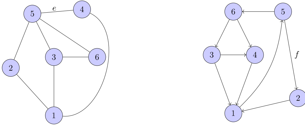
Σχήμα 7: (α) Ένα μη κατευθυνόμενο γράφημα και (β) ένα κατευθυνόμενο γράφημα.
