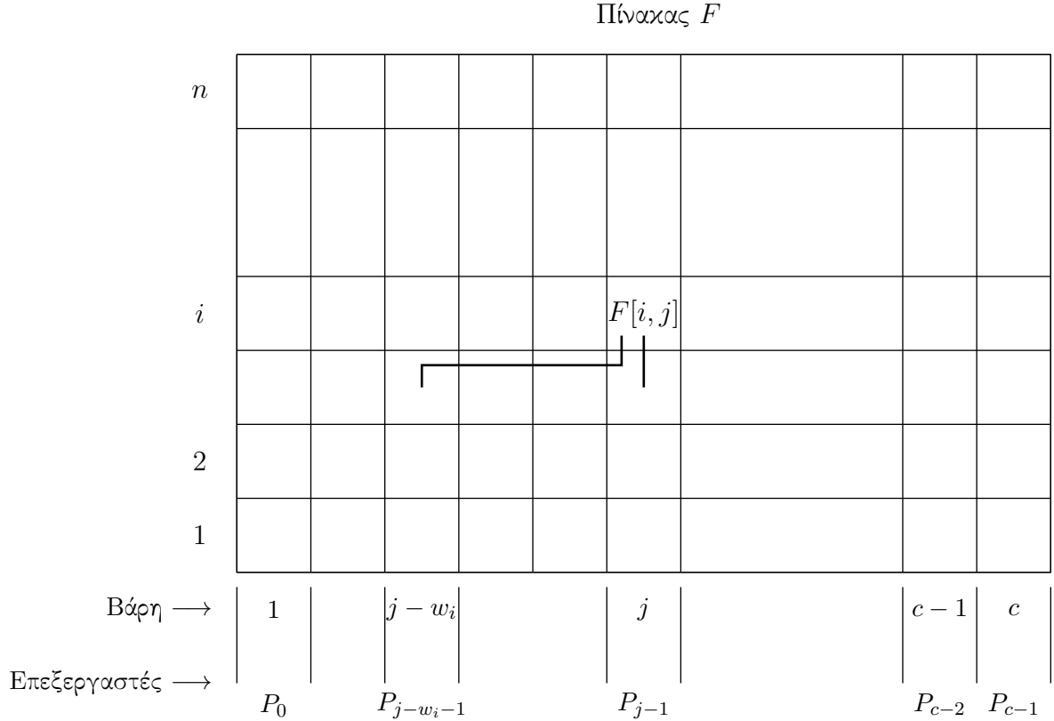
Σχήμα 36: Υπολογισμός καταχωρίσεων του πίνακα F για το πρόβλημα σακιδίου 0/1. Ο υπολογισμός της καταχώρισης F[i, j] απαιτεί επικοινωνία με επεξεργαστές που περιέχουν τις καταχωρίσεις F[i - 1, j] και F[i - 1, j - w_i] .
