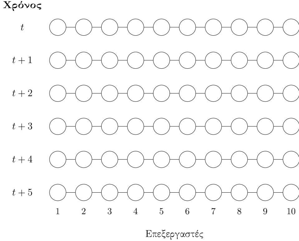
Σχήμα 43: Πρωτόκολλο επικοινωνίας που ακολουθείται στη υλοποίηση σωλήνωσης κατά μπλοκ σκακιέρας του αλγορίθμου του Floyd. Υποθέτουμε ότι ο επεξεργαστής 4 τη χρονική στιγμή t έχει μόλις υπολογίσει ένα τμήμα της k -οστής στήλης του πίνακα D^{(k-1)} . Το αποστέλλει στους επεξεργαστές 3 και 5. Αυτοί οι επεξεργαστές λαμβάνουν το τμήμα τη χρονική στιγμή t+1 (όπου η μονάδα χρόνου είναι ο χρόνος που χρειάζεται ένα τμήμα πίνακα για να διανύσει τον σύνδεσμο επικοινωνίας μεταξύ γειτονικών επεξεργαστών). Ομοίως, οι επεξεργαστές που απέχουν περισσότερο από τον επεξεργαστή 4 λαμβάνουν το τμήμα αργότερα. Ο επεξεργαστής 1 (στο όριο του πλέγματος) δεν προωθεί το τμήμα μετά την παραλαβή του.
