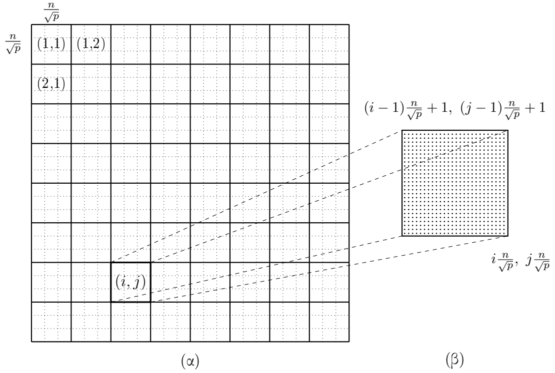
Σχήμα 38: (α) Ο πίνακας D^{(k)} διαμερισμένος με αντιστοίχιση σε μπλοκ σκακιέρας σε \sqrt{p} \times \sqrt{p} υπομπλοκ, και (β) το τετραγωνικό υπομπλοκ του D^{(k)} που ανατίθεται στον επεξεργαστή P_{i,j} .
