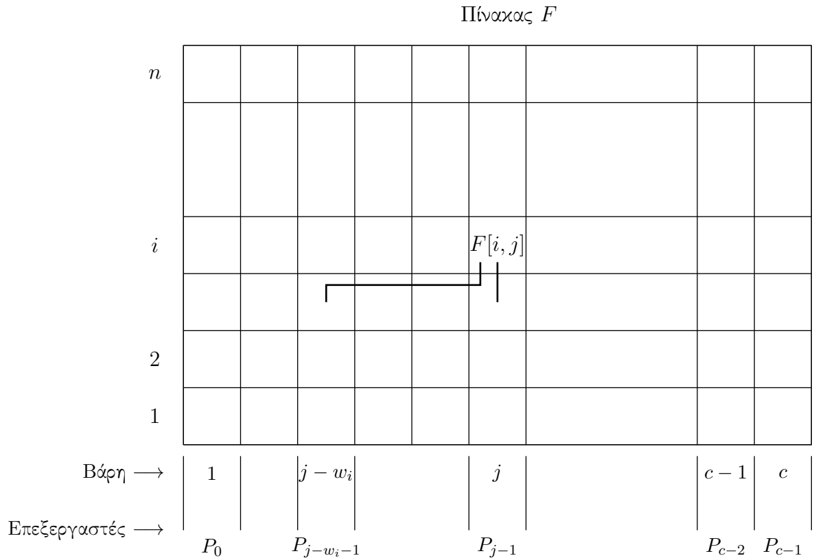
Σχήμα 55: Υπολογισμός καταχωρίσεων του πίνακα F για το πρόβλημα σακιδίου 0/1. Ο υπολογισμός της καταχώρισης F[i, j] απαιτεί επικοινωνία με επεξεργαστές που περιέχουν τις καταχωρίσεις F[i - 1, j] και F[i - 1, j - w_i] .
