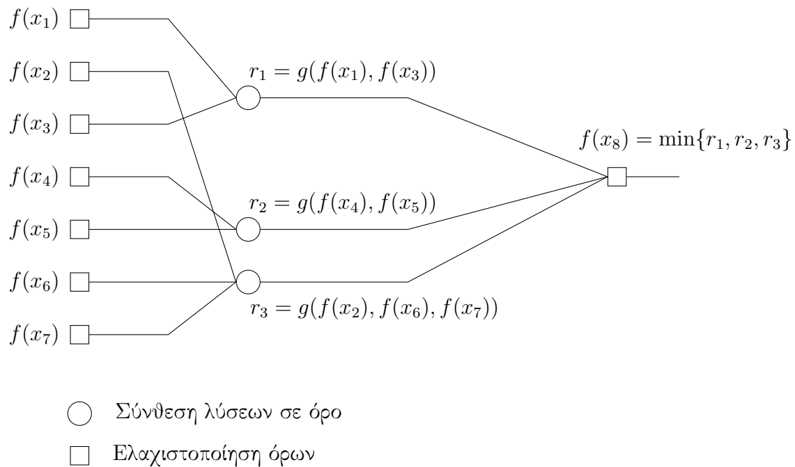
Σχήμα 53: Ο υπολογισμός και η σύνθεση λύσεων υποπροβλημάτων για την επίλυση του προβλήματος f(x_8) .
