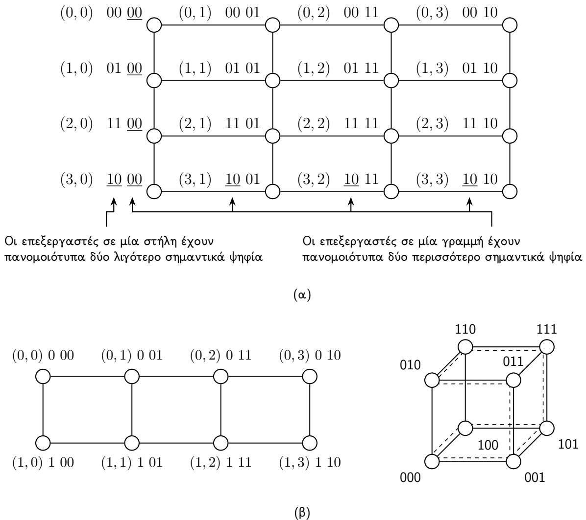
Σχήμα 23: (α) Ένα πλέγμα 4 \times 4 που απεικονίζει την αντιστοίχιση των επεξεργαστών του πλέγματος σε επεξεργαστές ενός τετραδιάστατου υπερκύβου και (β) ένα πλέγμα επεξεργαστών 2 \times 4 εμφυτευμένο σε έναν τριδιάστατο υπερκύβο.
