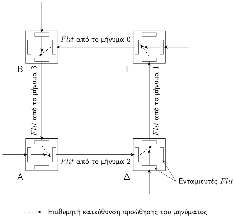
Σχήμα 27: Ένα παράδειγμα αδιεξόδου σε ένα δίκτυο δρομολόγησης σκληροειδούς προώθησης.
