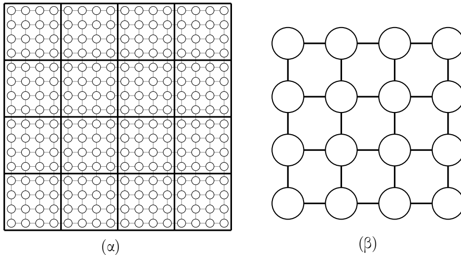
Σχήμα 51: Απεικόνιση του γραφήματος πλέγματος (α) σε ένα πλέγμα (β) χρησιμοποιώντας την απεικόνιση μπλοκ σκακιέρας. Σε αυτό το παράδειγμα, n = 16 και \sqrt{p} = 4 . Οι σκιασμένες κορυφές απεικονίζονται στον σκιασμένο επεξεργαστή.
