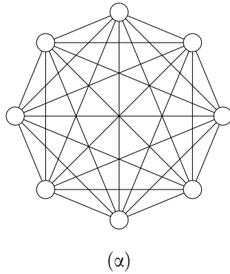
Σχήμα 14: Ένα πλήρως συνδεδεμένο δίκτυο οκτώ επεξεργαστών (α) και ένα συνδεδεμένο δίκτυο αστέρα εννέα επεξεργαστών (β).
