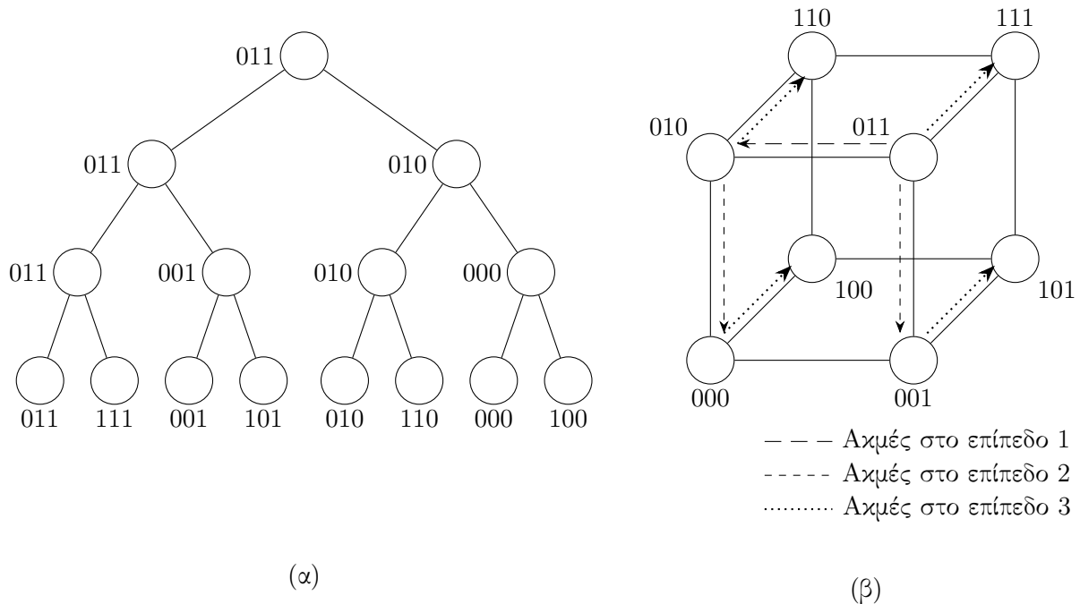
Σχήμα 24: Ένα δέντρο με ρίζα τον επεξεργαστή 011 (=3) εμφυτευμένο σε έναν τριδιάστατο υπερκύβο: (α) η οργάνωση του δέντρου με ρίζα τον επεξεργαστή 011, και (β) το δέντρο εμφυτευμένο σε έναν τριδιάστατο υπερκύβο.
