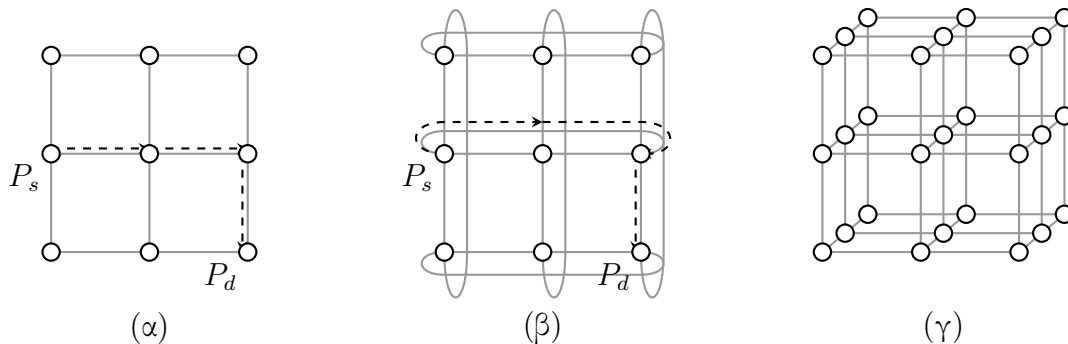
Σχήμα 16: (α) Ένα διδιάστατο πλέγμα με παράδειγμα δρομολόγησης ενός μηνύματος από τον επεξεργαστή P_s στον επεξεργαστή P_d . (β) Ένα διδιάστατο πλέγμα με σύνδεση αναδίπλωσης με παράδειγμα δρομολόγησης ενός μηνύματος από τον επεξεργαστή P_s στον επεξεργαστή P_d . (γ) Ένα τριδιάστατο πλέγμα.
