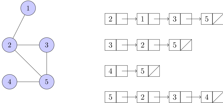
Σχήμα 31: Ένα μη κατευθυνόμενο γράφημα και η αναπαράστασή του με λίστα γειτνίασης.
