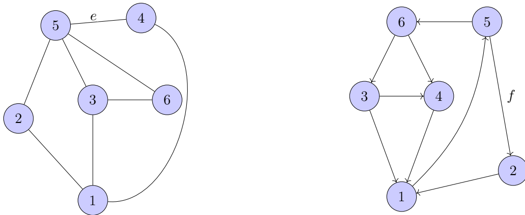
Σχήμα 29: (α) Ένα μη κατευθυνόμενο γράφημα και (β) ένα κατευθυνόμενο γράφημα.
