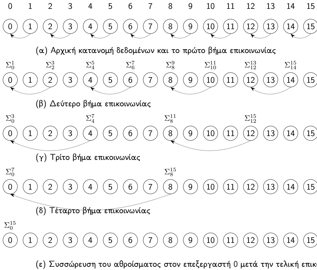
Σχήμα 28: Υπολογισμός του αθροίσματος 16 αριθμών σε έναν υπερκύβο 16 επεξεργαστών. Το \Sigma_i^j συμβολίζει το άθροισμα των αριθμών με διαδοχικές ετικέτες από i έως j .
