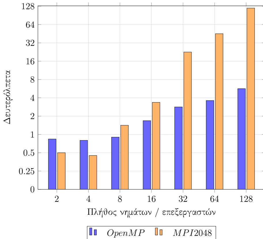
Σχήμα 37: Διαφορετικά νήματα/επεξεργαστές για την υλοποίηση OpenMP και MPI σε γράφημα με 2048 κορυφές
