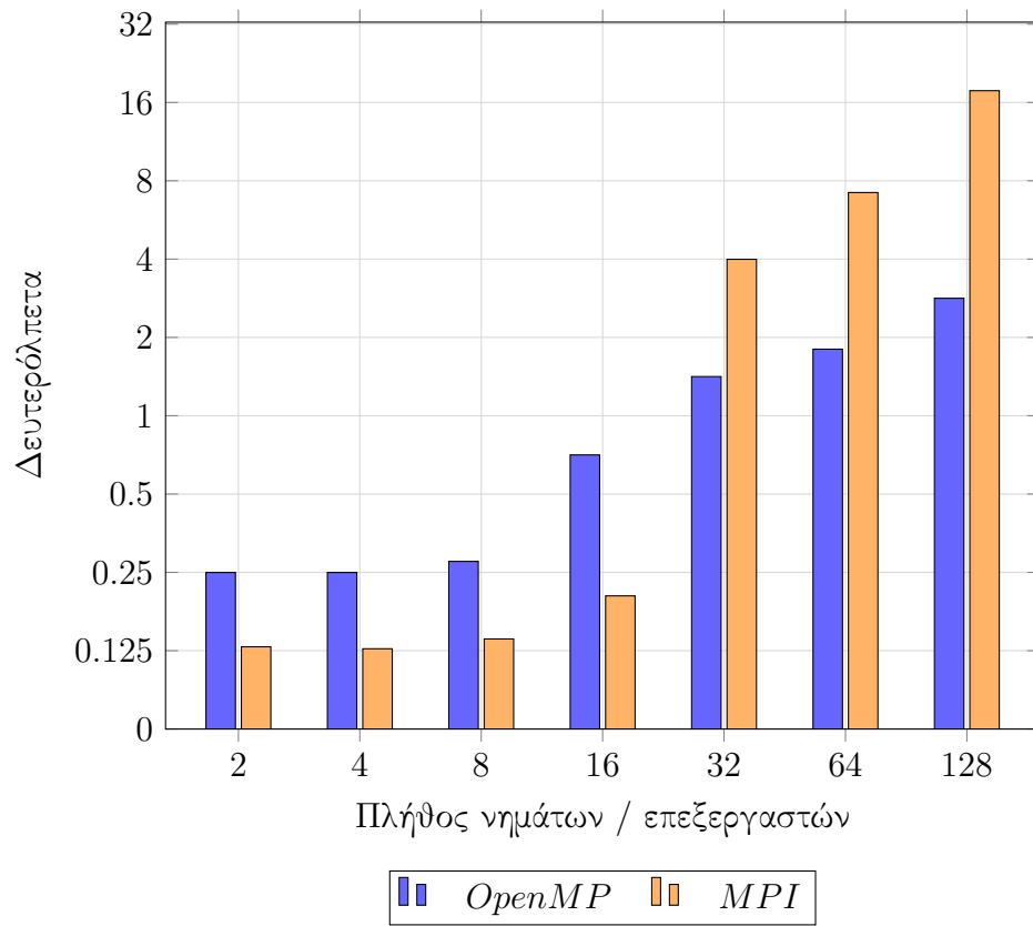
Σχήμα 37: Διαφορετικά νήματα/επεξεργαστές για την υλοποίηση OpenMP και MPI σε γράφημα με 1024 κορυφές
