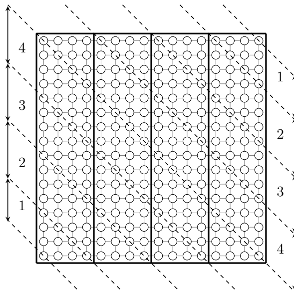
Σχήμα 55: Ο αριθμός των απασχολημένων επεξεργαστών αυξάνεται καθώς το κύμα διαδίδεται μέσα από το γράφημα πλέγματος.
