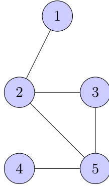
Σχήμα 31: Ένα μη κατευθυνόμενο γράφημα και η αναπαράστασή του με πίνακα γειτνίασης.
