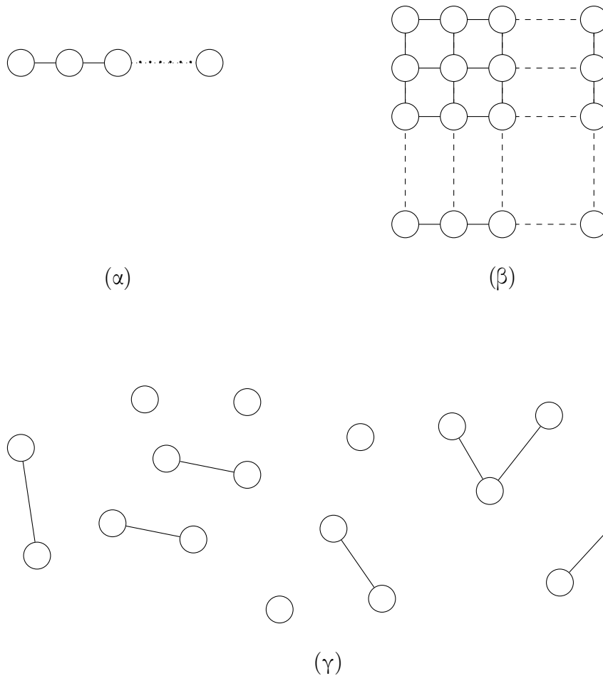
Σχήμα 48: Παραδείγματα αραιών γραφημάτων: (α) ένα γραμμικό γράφημα, στον οποίο κάθε κορυφή έχει δύο προσπίπτουσες ακμές, (β) ένα γράφημα πλέγματος, στον οποίο κάθε κορυφή έχει τέσσερις γειτονικές κορυφές και (γ) τυχαίο αραιό γράφημα.
