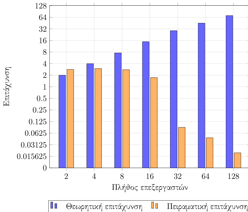
Σχήμα 39: Η σύγκριση της θεωρητικής επιτάχυνσης με την πειραματική επιτάχυνση για την υλοποίηση MPI για γράφημα 1024 κορυφών σε διαφορετικούς επεξεργαστές
