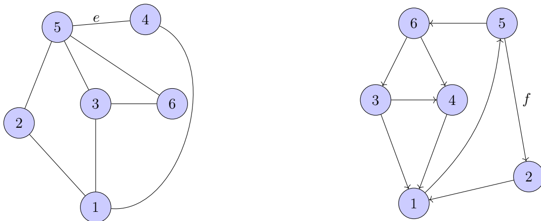
Σχήμα 30: (α) Ένα μη κατευθυνόμενο γράφημα και (β) ένα κατευθυνόμενο γράφημα.
