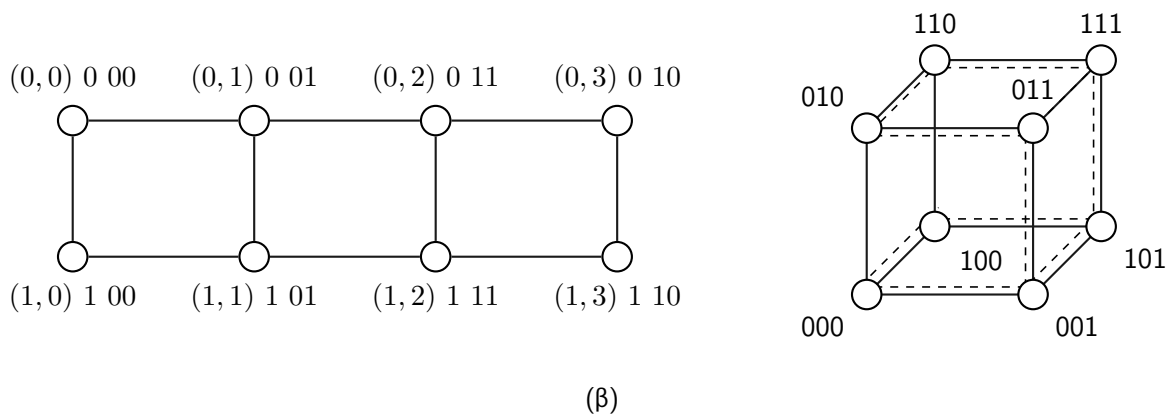
Σχήμα 23: (α) Ένα πλέγμα 4 \times 4 που απεικονίζει την αντιστοίχιση των επεξεργαστών του πλέγματος σε επεξεργαστές ενός τετραδιάστατου υπερκύβου και (β) ένα πλέγμα επεξεργαστών 2 \times 4 εμφυτευμένο σε έναν τριδιάστατο υπερκύβο.
