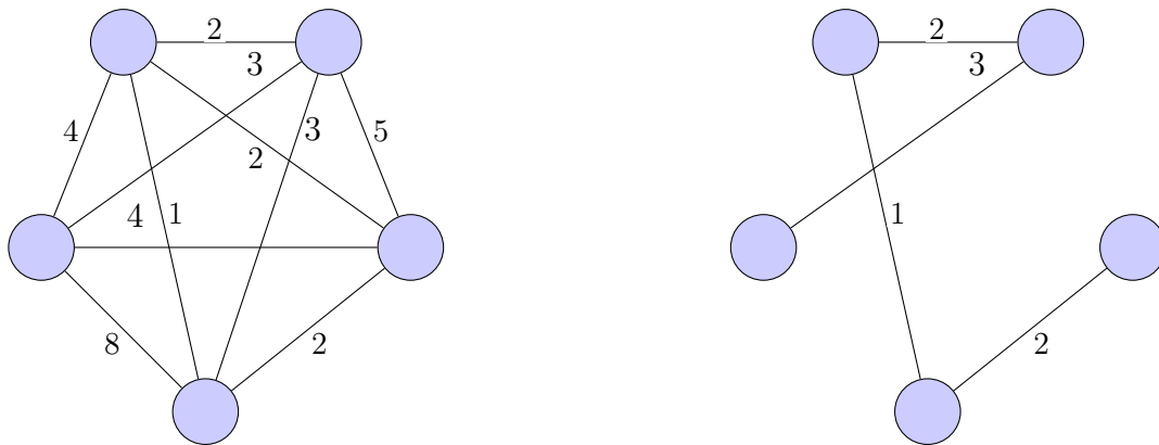
Σχήμα 33: Ένα μη κατευθυνόμενο γράφημα και το ελάχιστο δέντρο επικάλυψης του.
