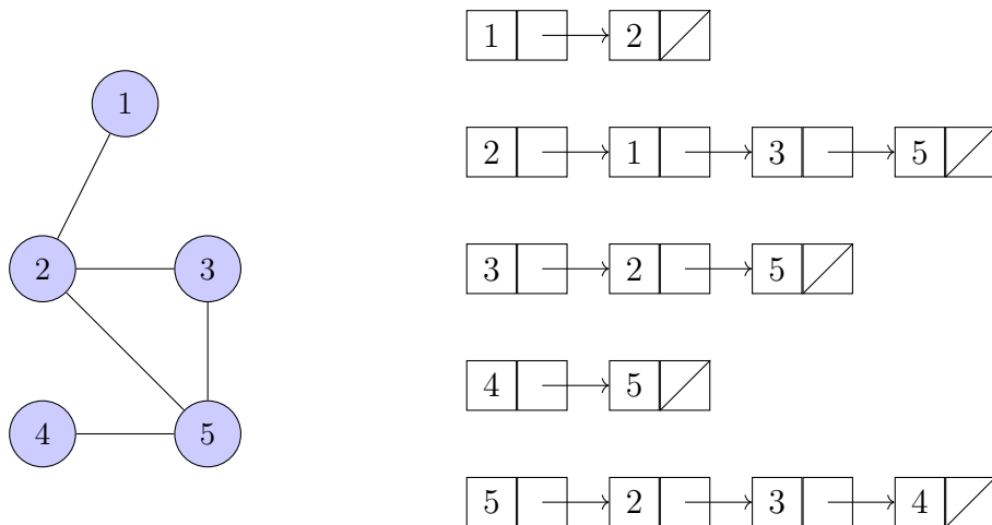
Σχήμα 32: Ένα μη κατευθυνόμενο γράφημα και η αναπαράσταση του με λίστα γειτνίασης.
