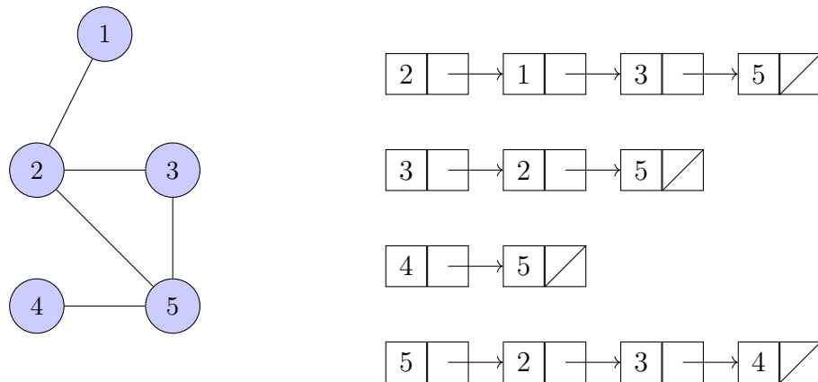
Σχήμα 31: Ένα μη κατευθυνόμενο γράφημα και η αναπαράσταση του με λίστα γειτνίασης.
