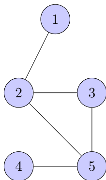
Σχήμα 2: Ένα μη κατευθυνόμενο γράφημα και η αναπαράσταση του με λίστα γειτνίασης.
