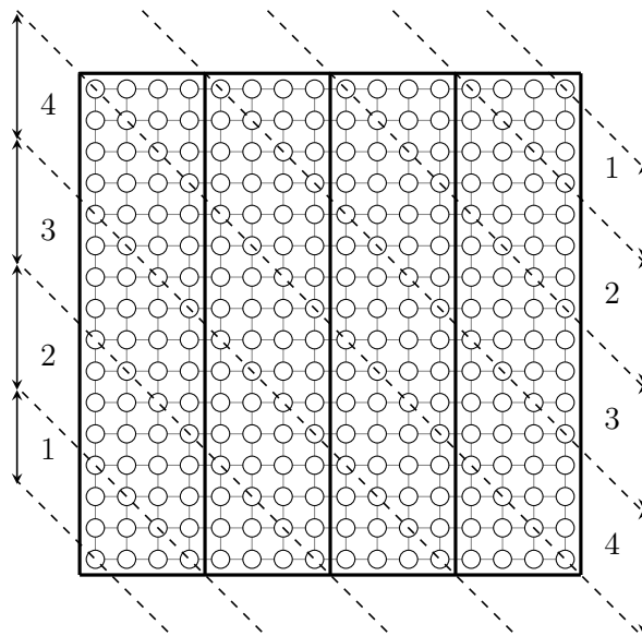
Σχήμα 46: Ο αριθμός των απασχολημένων επεξεργαστών αυξάνεται καθώς το κύμα διαδίδεται μέσα από το γράφημα πλέγματος.
