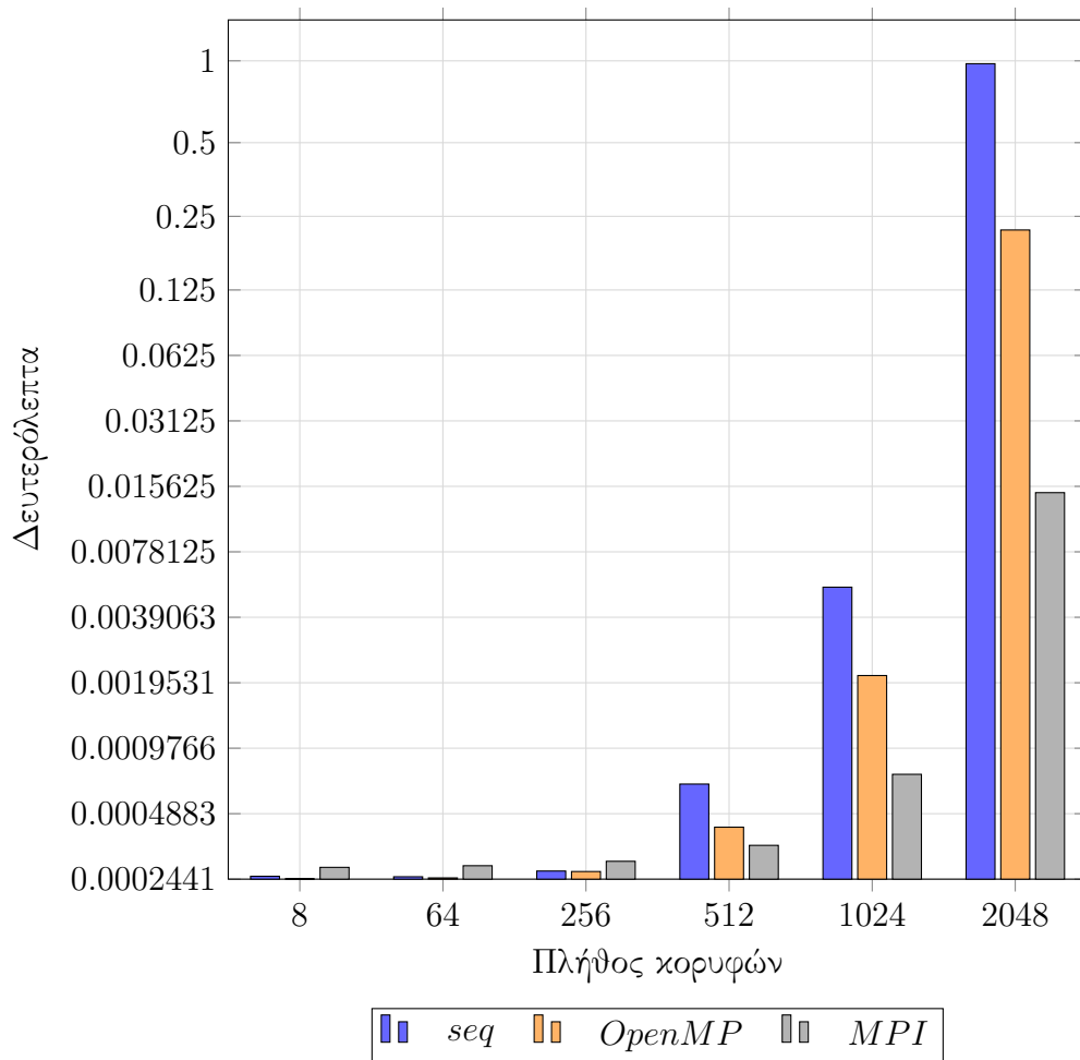
Σχήμα 7: Ο καλύτερος χρόνος εκτέλεσης για κάθε υλοποίηση σε διαφορετικά σύνολα δεδομένων
