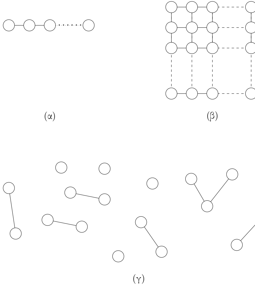
Σχήμα 22: Παραδείγματα αραιών γραφημάτων: (α) ένα γραμμικό γράφημα, στον οποίο κάθε κορυφή έχει δύο προσπίπτουσες ακμές, (β) ένα γράφημα πλέγματος, στον οποίο κάθε κορυφή έχει τέσσερις γειτονικές κορυφές και (γ) τυχαίο αραιό γράφημα.
