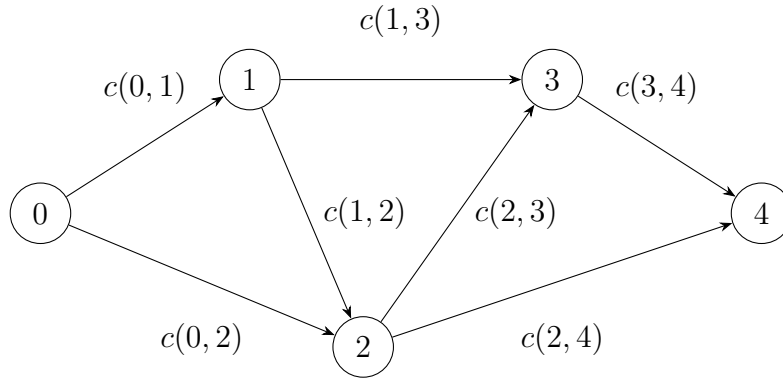
Σχήμα 30: Ένα γράφημα για το οποίο πρέπει να υπολογιστεί το συντομότερο μονοπάτι μεταξύ των κόμβων 0 και 4.
