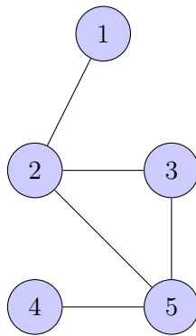
Σχήμα 5: Ένα μη κατευθυνόμενο γράφημα και η αναπαράσταση του με λίστα γειτνίασης.
