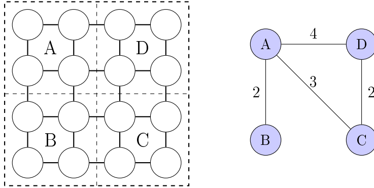
Σχήμα 15: Διαμέριση ενός πλέγματος \sqrt{p} \times \sqrt{p} σε n υποπλέγματα, καθένα με μέγεθος \sqrt{p/n} \times \sqrt{p/n} . Στο παράδειγμα αυτό, p = 16 και n = 4 . Κάθε ένα από τα πλέγματα μεγέθους \sqrt{p/n} \times \sqrt{p/n} = 2 \times 2 επιλύει το πρόβλημα των συντομότερων διαδρομών μονής πηγής για μια δοσμένη κορυφή πηγής. Στο παράδειγμα αυτό, κάθε υποπλέγμα επισημαίνεται από την κορυφή πηγής του αντίστοιχου αλγορίθμου μονής πηγής.
