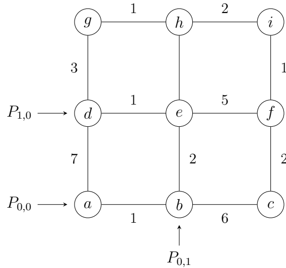
Σχήμα 28: Ένα γράφημα πλέγματος.
