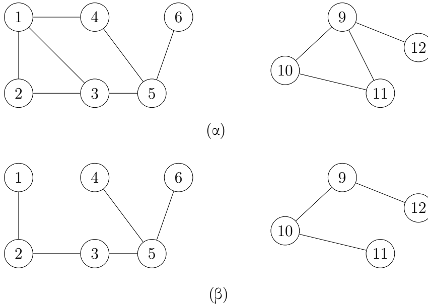
Σχήμα 24: Το μέρος (β) είναι ένα δάσος πρώτα κατά βάθος που προκύπτει από διάσχιση πρώτα κατά βάθος του γραφήματος στο μέρος (α). Κάθε ένα από αυτά τα δέντρα είναι μια συνεκτική συνιστώσα του γραφήματος στο μέρος (α).
