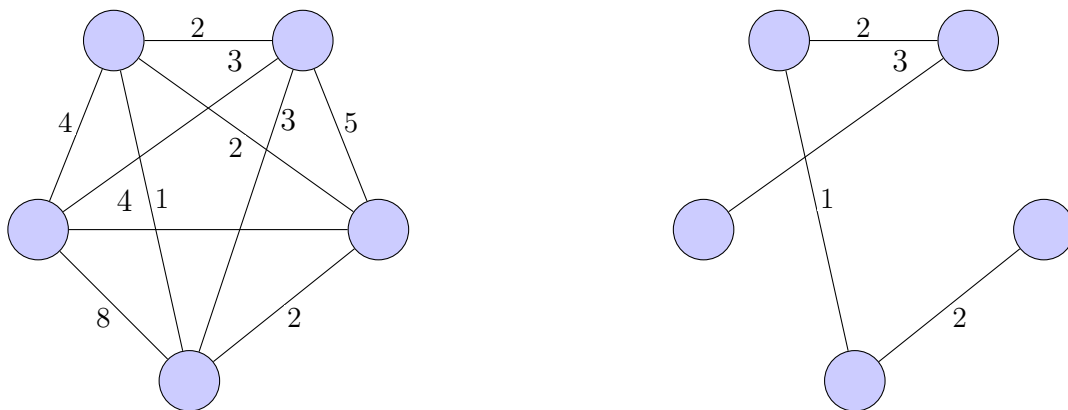
Σχήμα 11: Ένα μη κατευθυνόμενο γράφημα και το ελάχιστο δέντρο επικάλυψης του.
