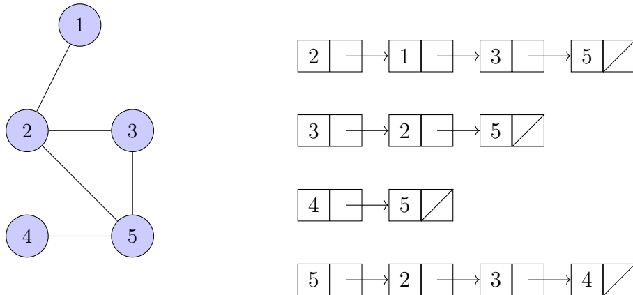
Σχήμα 10: Ένα μη κατευθυνόμενο γράφημα και η αναπαράσταση του με λίστα γειτνίασης.
