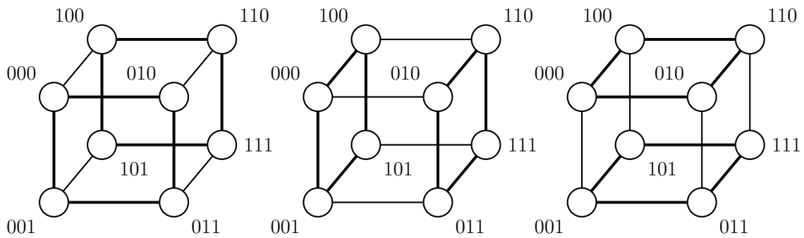
Σχήμα 20: Τρεις διακριτές διαμερίσεις ενός τρισδιάστατου υπερκύβου σε δύο δισδιάστατους κύβους. Οι σύνδεσμοι που συνδέουν επεξεργαστές μέσα σε μία διαμέριση υποδεικνύονται με έντονες γραμμές.
