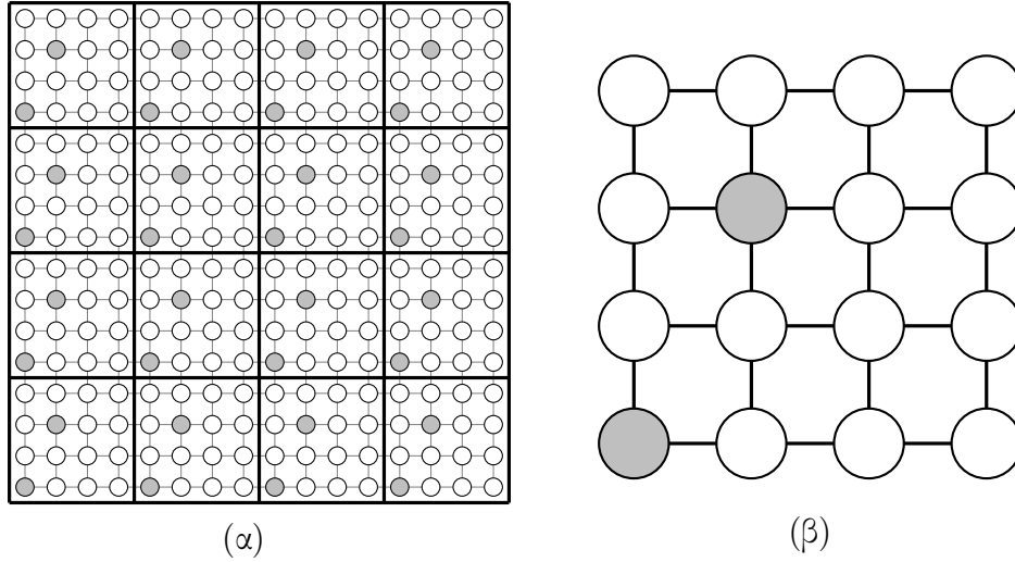
Σχήμα 24: Απεικόνιση του γραφήματος πλέγματος (α) σε ένα πλέγμα (β) χρησιμοποιώντας την κυκλική απεικόνιση σκακιέρας. Σε αυτό το παράδειγμα, n = 16 και \sqrt{p} = 4 . Οι σκιασμένες κορυφές απεικονίζονται στους αντίστοιχους σκιασμένους επεξεργαστές πλέγματος.
