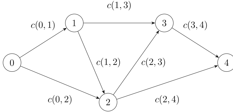
Σχήμα 27: Ένα γράφημα για το οποίο πρέπει να υπολογιστεί το συντομότερο μονοπάτι μεταξύ των κόμβων 0 και 4.
