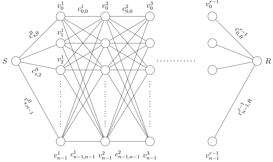
Σχήμα 29: Ένα παράδειγμα σειριακής μοναδικής υλοποίησης \Delta\Pi για την εύρεση του συντομότερου μονοπατιού σε ένα γράφημα του οποίου οι κόμβοι μπορούν να οργανωθούν σε επίπεδα.
