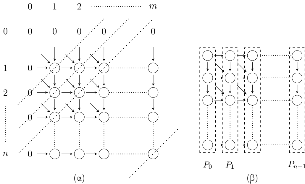
Σχήμα 52: (α) Υπολογισμός καταχωρίσεων του πίνακα F για το πρόβλημα μέγιστης κοινής υπακολουθίας. Ο υπολογισμός προχωρά κατά μήκος των διακεκομμένων διαγώνιων γραμμών. (β) Αντιστοίχιση στοιχείων του πίνακα σε επεξεργαστές.
