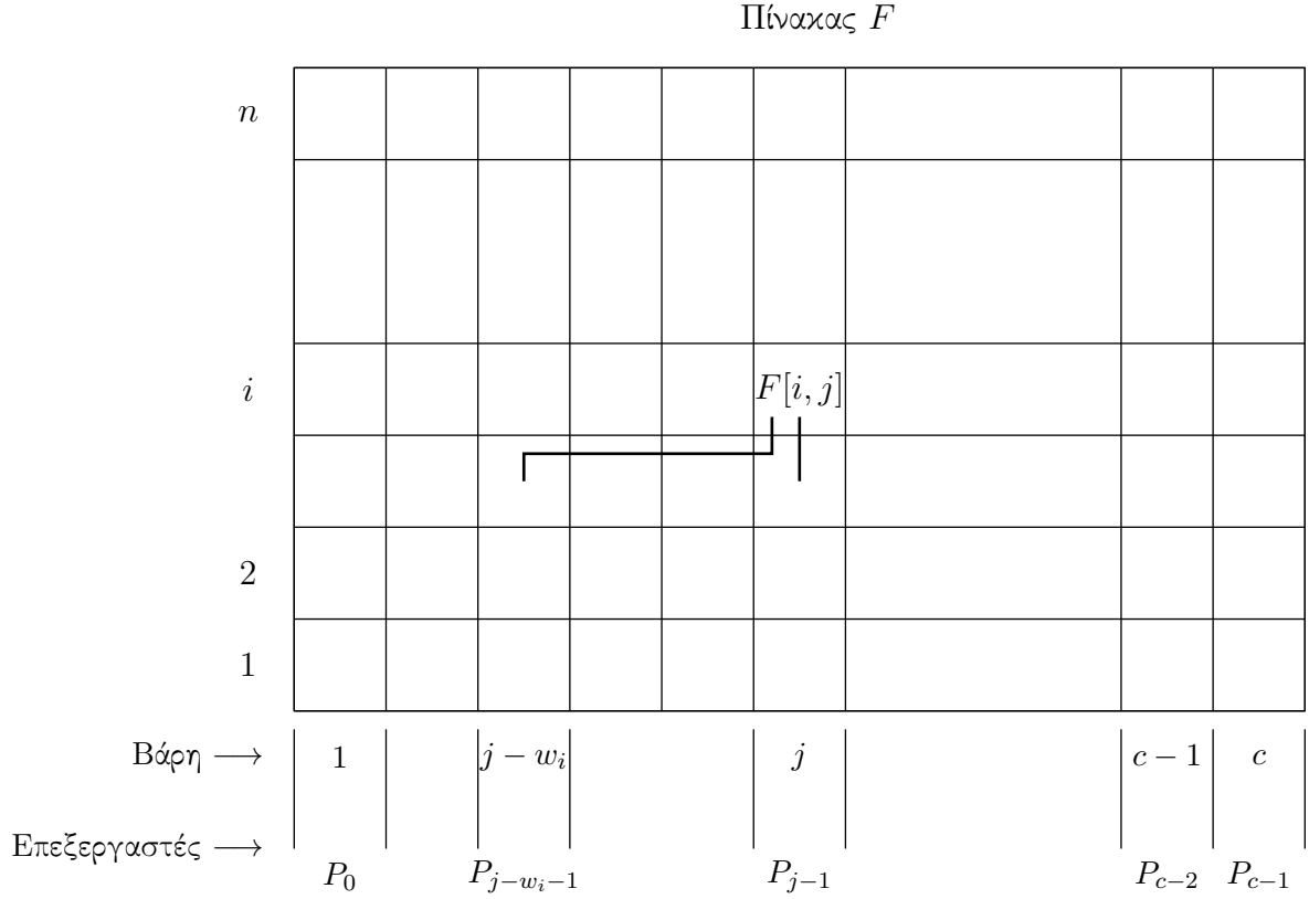
Σχήμα 51: Υπολογισμός καταχωρίσεων του πίνακα F για το πρόβλημα σαχιδίου 0/1. Ο υπολογισμός της καταχώρισης F[i, j] απαιτεί επικοινωνία με επεξεργαστές που περιέχουν τις καταχωρίσεις F[i - 1, j] και F[i - 1, j - w_i] .
