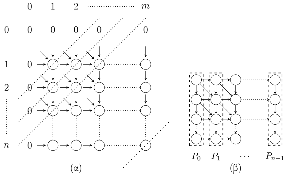
Σχήμα 31: (α) Υπολογισμός καταχωρίσεων του πίνακα F για το πρόβλημα μεγαλύτερης κοινής υπακολουθίας. Ο υπολογισμός προχωρά κατά μήκος των διακεκομμένων διαγώνιων γραμμών. (β) Αντιστοίχιση στοιχείων του πίνακα σε επεξεργαστές.
