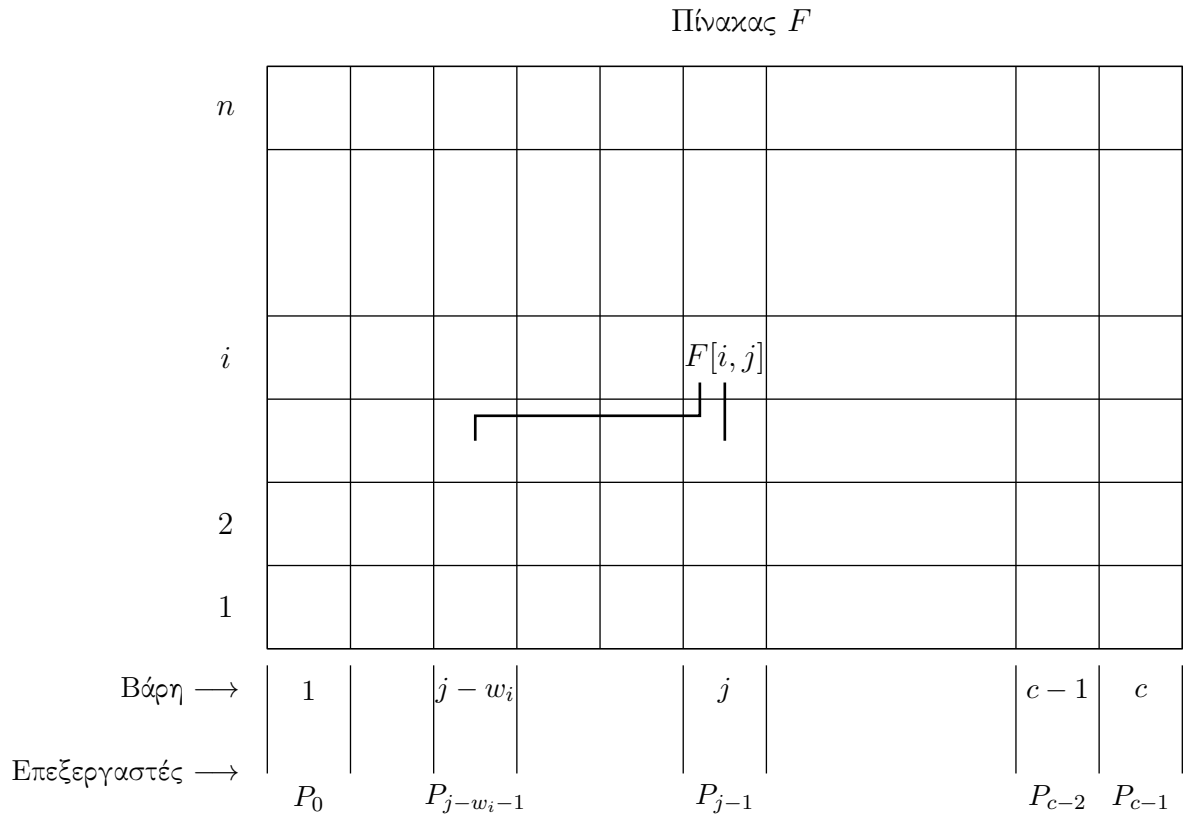
Σχήμα 30: Υπολογισμός καταχωρίσεων του πίνακα F για το πρόβλημα σακιδίου 0/1. Ο υπολογισμός της καταχώρισης F[i, j] απαιτεί επικοινωνία με επεξεργαστές που περιέχουν τις καταχωρίσεις F[i - 1, j] και F[i - 1, j - w_i] .
