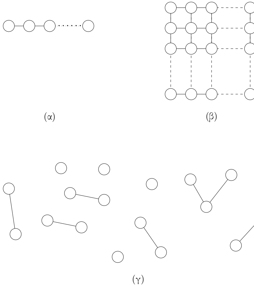
Σχήμα 28: Παραδείγματα αραιών γραφημάτων: (α) ένα γραμμικό γράφημα, στον οποίο κάθε κορυφή έχει δύο προσπίπτουσες ακμές, (β) ένα γράφημα πλέγματος, στον οποίο κάθε κορυφή έχει τέσσερις γειτονικές κορυφές και (γ) τυχαίο αραιό γράφημα.
