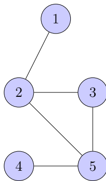
Σχήμα 11: Ένα μη κατευθυνόμενο γράφημα και η αναπαράσταση του με πίνακα γειτνίασης.
