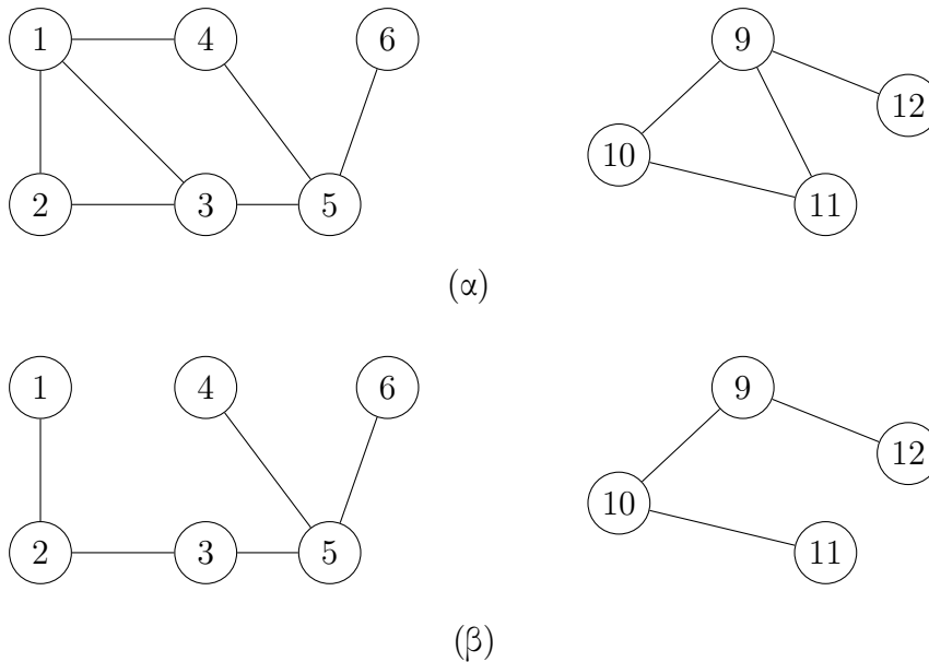
Σχήμα 26: Το μέρος (β) είναι ένα δάσος πρώτα κατά βάθος που προκύπτει από διάσχιση πρώτα κατά βάθος του γραφήματος στο μέρος (α). Κάθε ένα από αυτά τα δέντρα είναι μια συνεκτική συνιστώσα του γραφήματος στο μέρος (α).
