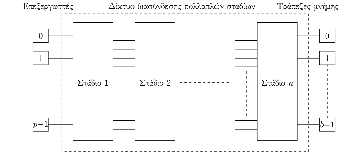
Σχήμα 8: Η σχηματική αναπαράσταση ενός τυπικού δικτύου διασύνδεσης πολλαπλών σταδίων.
