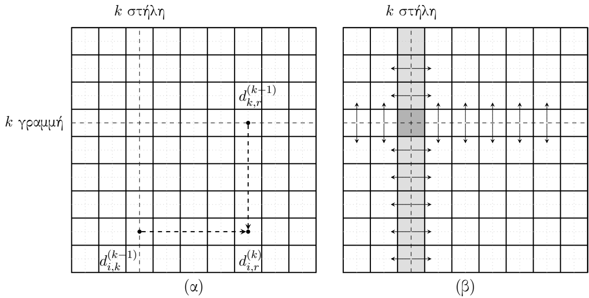
Σχήμα 23: (α) Μοτίβα επικοινωνίας που χρησιμοποιούνται στην αντιστοίχιση σε μπλοκ σκακιέρας. Κατά τον υπολογισμό του d_{i,j}^{(k)} , πληροφορίες πρέπει να αποσταλούν στον επιλεγμένο επεξεργαστή από δύο άλλους επεξεργαστές κατά μήκος της ίδιας γραμμής και στήλης. (β) Η γραμμή και η στήλη από \sqrt{p} επεξεργαστές που περιέχουν την k -οστή γραμμή και στήλη, τις αποστέλλουν κατά μήκος των στηλών και γραμμών επεξεργαστών.
