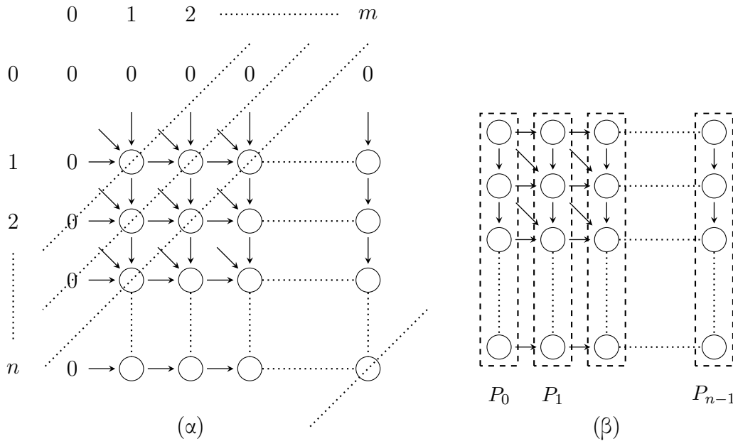
Σχήμα 40: (α) Υπολογισμός καταχωρίσεων του πίνακα F για το πρόβλημα μέγιστης κοινής υπακολουθίας. Ο υπολογισμός προχωρά κατά μήκος των διακεκομμένων διαγώνιων γραμμών. (β) Αντιστοίχιση στοιχείων του πίνακα σε επεξεργαστές.
