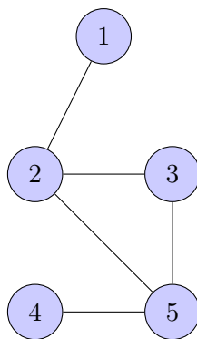
Σχήμα 22: (α) Ένα μη κατευθυνόμενο γράφημα και (β) ένα κατευθυνόμενο γράφημα.
